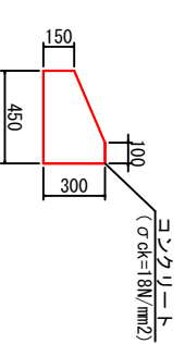
基礎工 S=1:20
