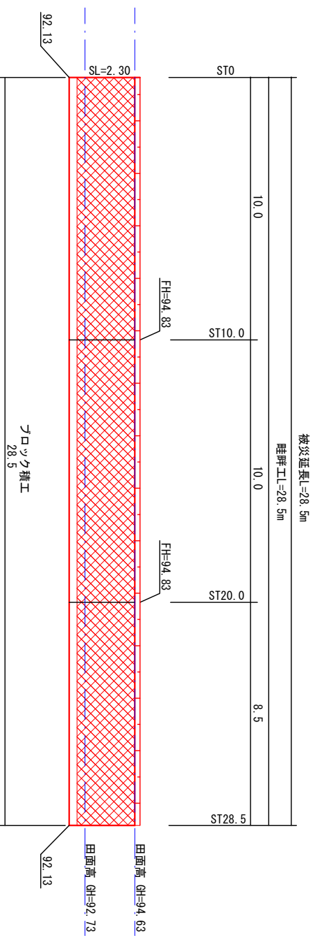
展開図 S=1:100
