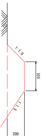
畦畔築立 縮尺=1:20
