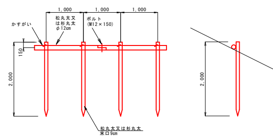
一本胴木 S=1:50
