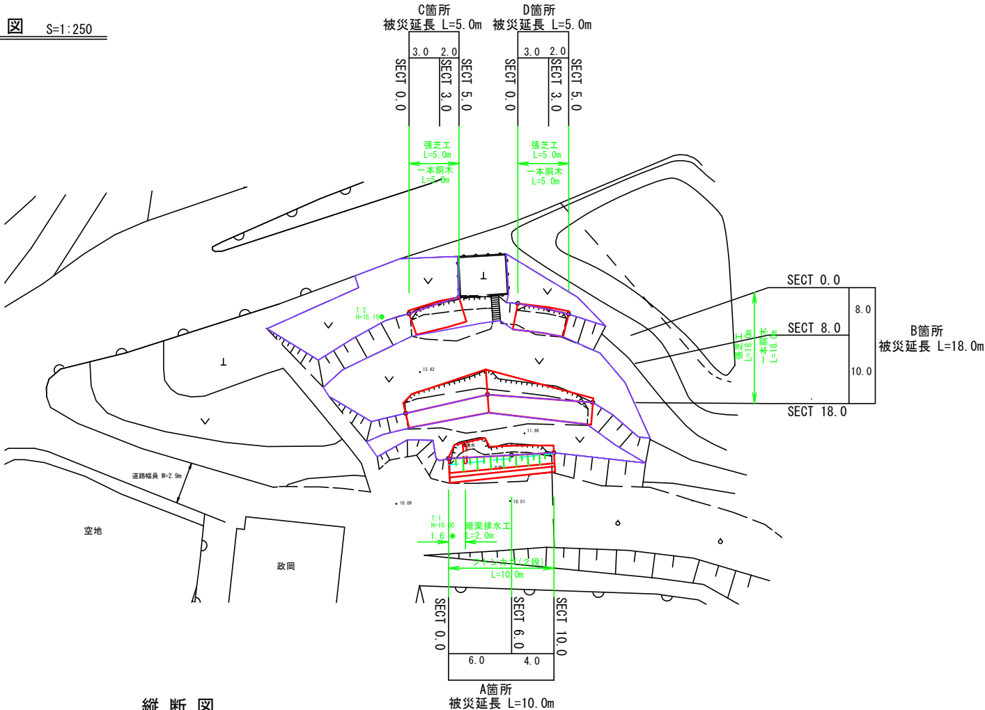
縦断図
