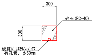
暗渠排水工 S=1:20
