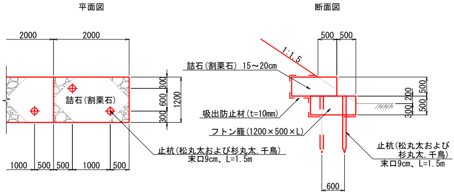
フトン籠 S=1:50
