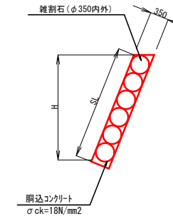
すり付け工 (練石積) S=1:50
