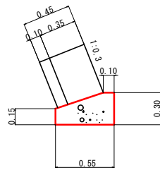
基礎工 S=1:25
