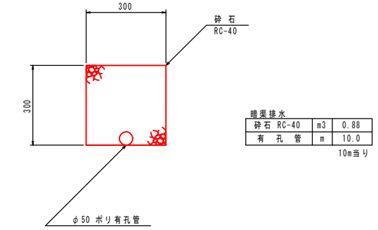
暗渠排水 縮尺=1:10
