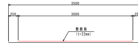
縮尺=1:30
