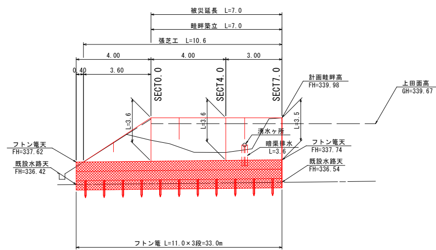
展開図 S=1:100
