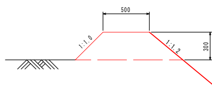
畦畔築立 (B箇所) 縮尺=1:20
