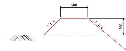
畦畔築立 (A箇所) 縮尺=1:20
