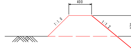
畦畔築立 (C箇所) 縮尺=1:20
