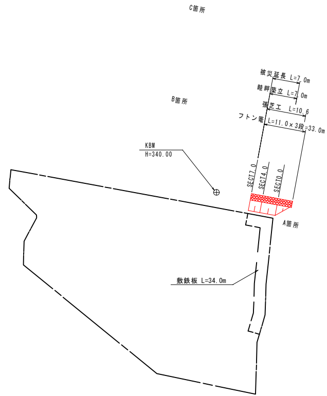
計画平面図 S=1:500
