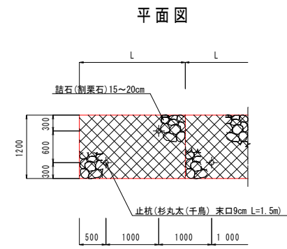
フトン籠 縮尺=1:50
