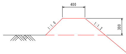
畦畔築立 縮尺=1:20
