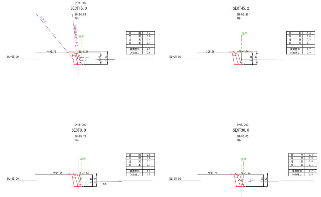
横断面 S=1:100
