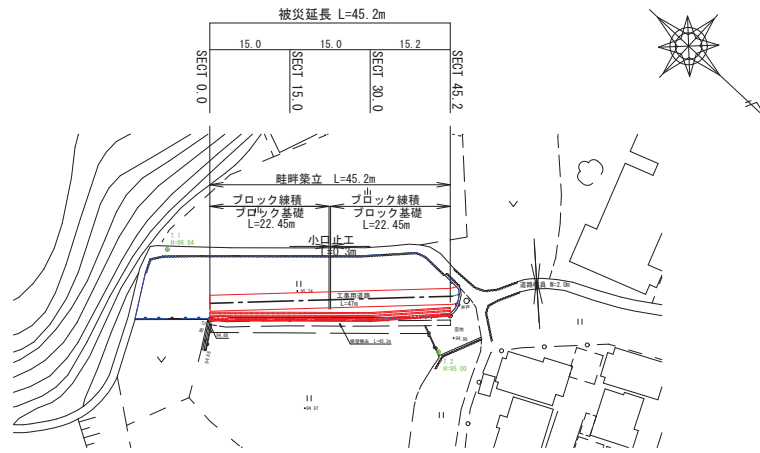
平面図 S=1:500
