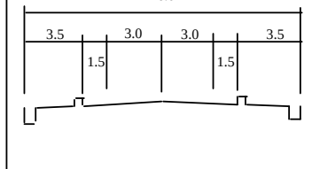
標準横断面図
