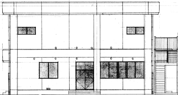
西 面 姿 図 1/100
