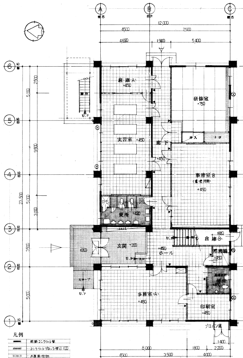
1 階平面図 1/100
