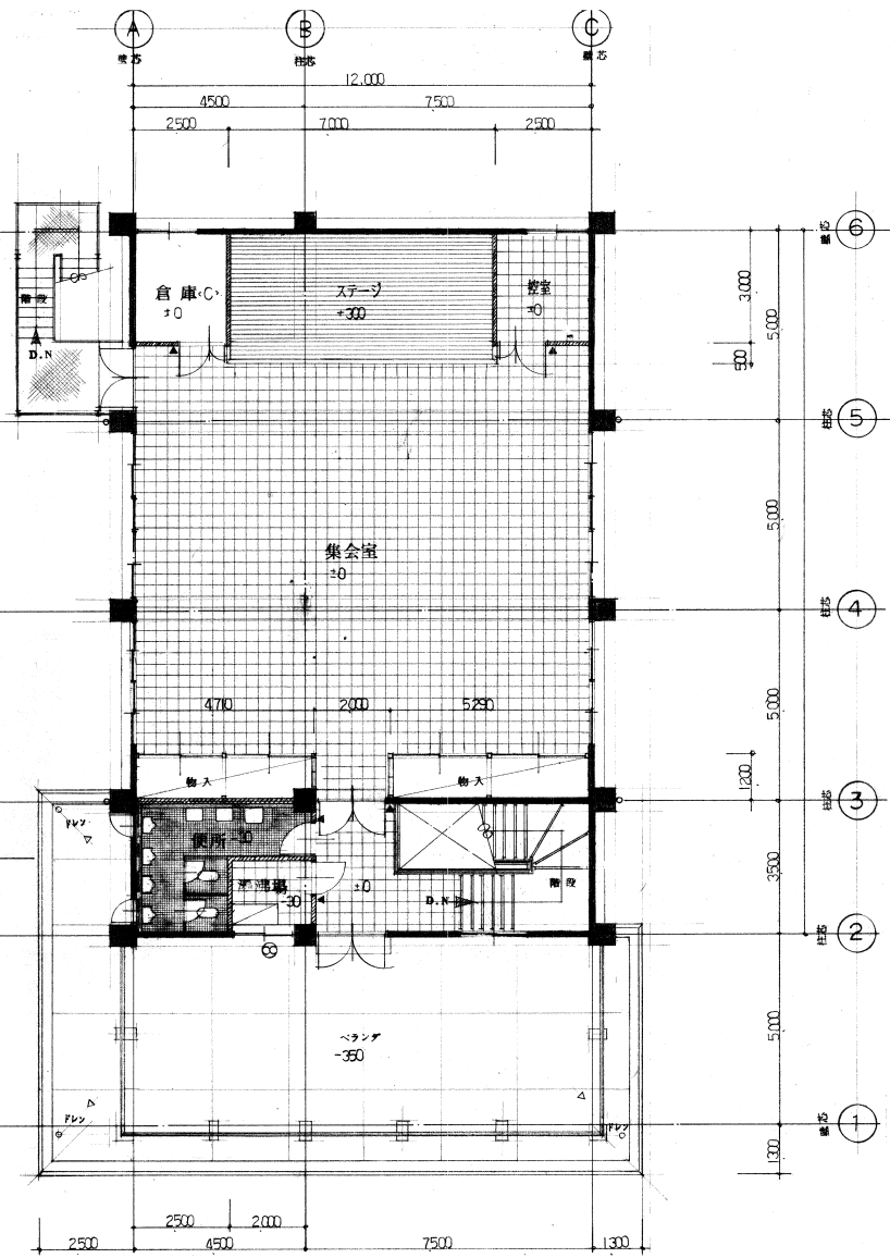
2 階平面図 1/100
