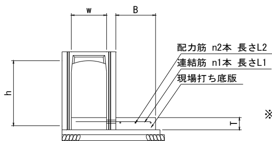
自由勾配側溝 寸法表
