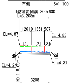
1号水路展開図
