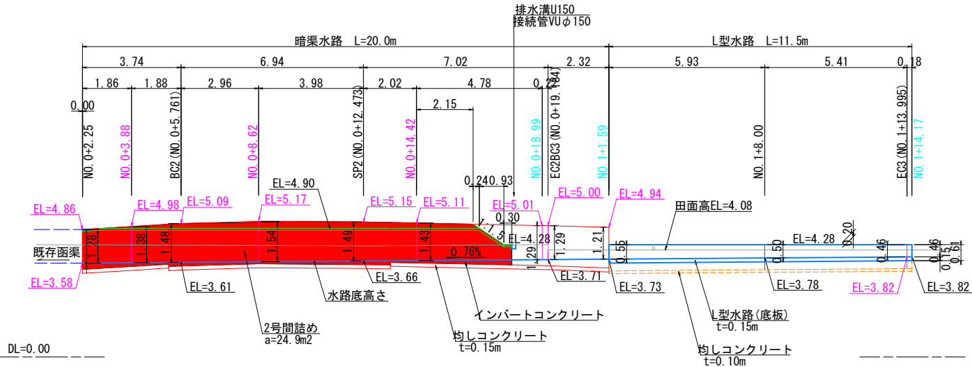
排水施設展開図
