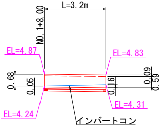
1号水路展開図
