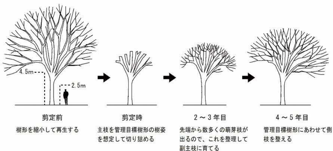
図 街路樹の仕立て直しの手法
