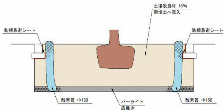
図 植栽基盤改良例
