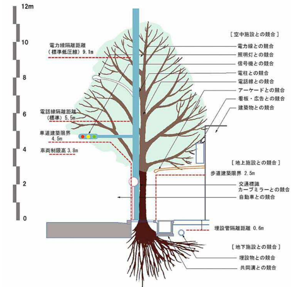
図 車道部・歩道部の建築限界
