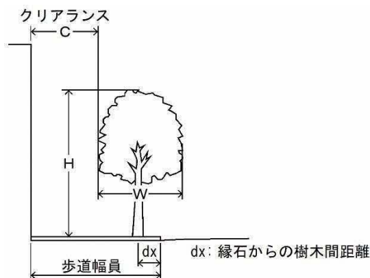
図表 枝張りの最大値（B）の算出
