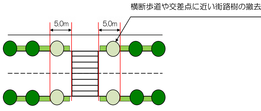
図 視認性確保の例
