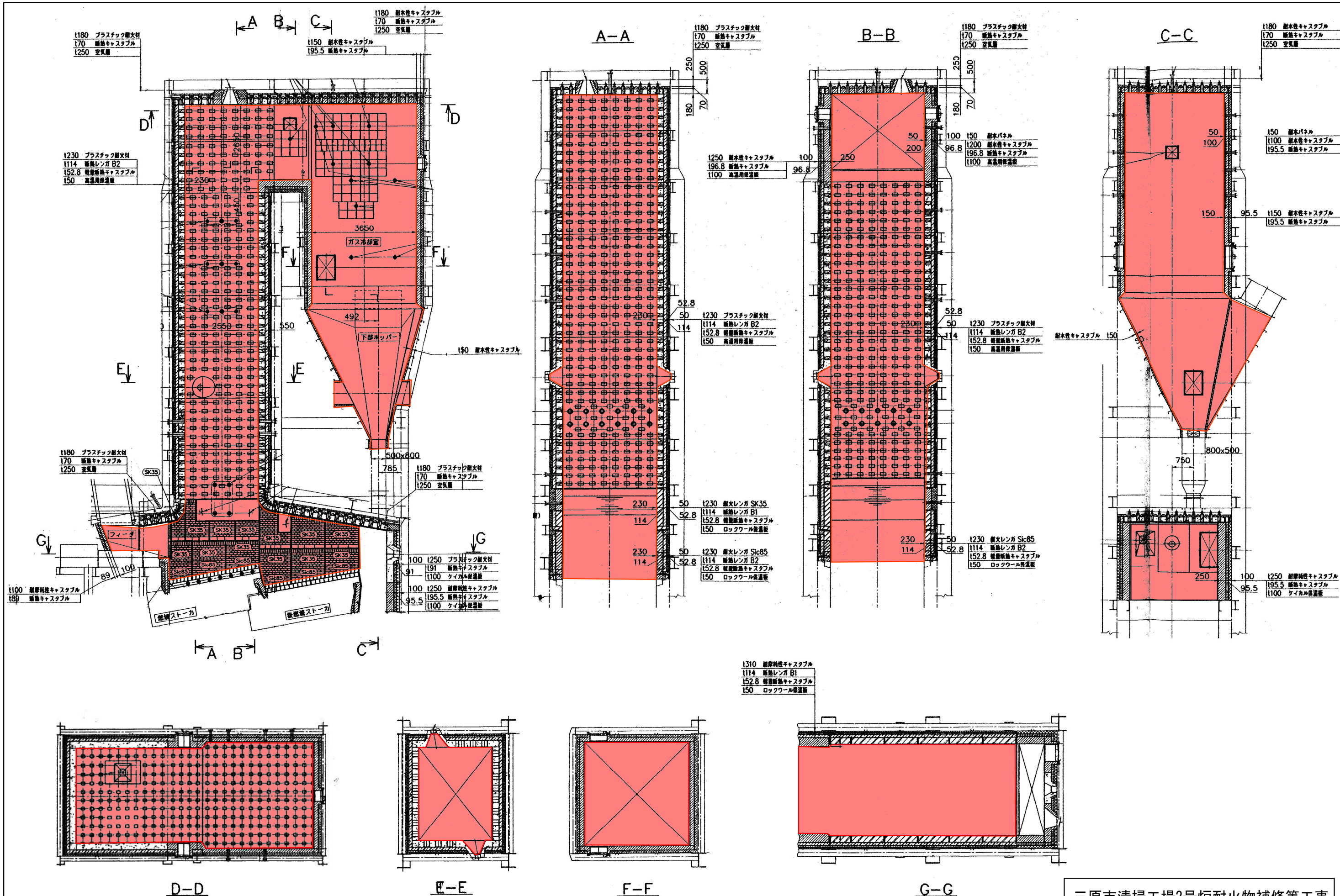
三原市清掃工場2号炉耐火物補修等工事 クリンカー除去範囲図
