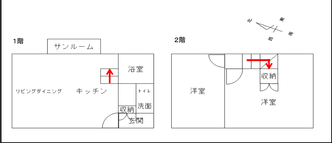
間取図
