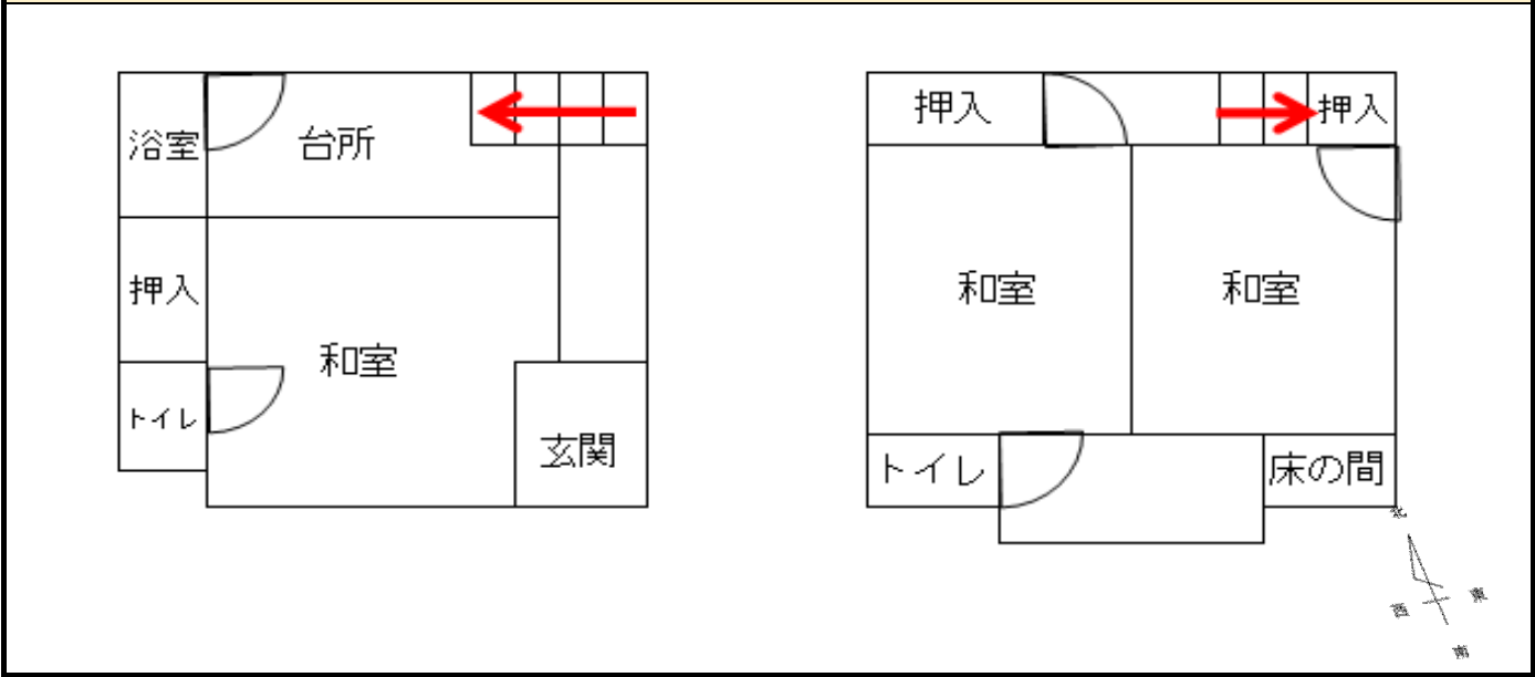
間取図
