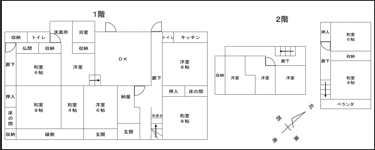
間取図
