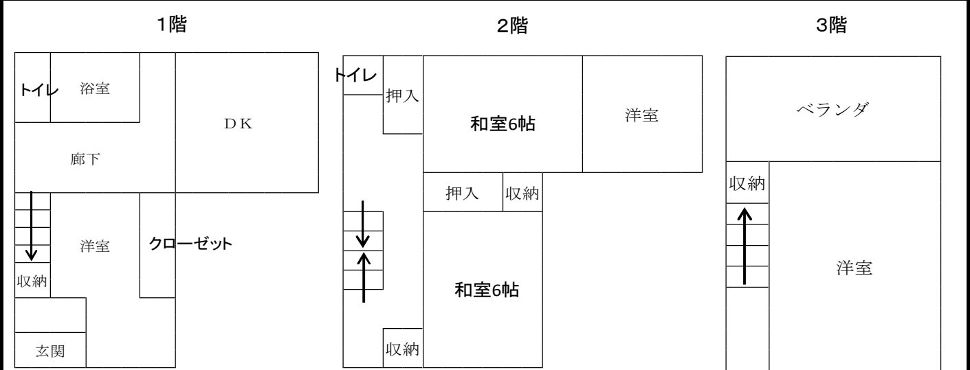
間取図
