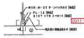
吊り材 詳細図 1/20
