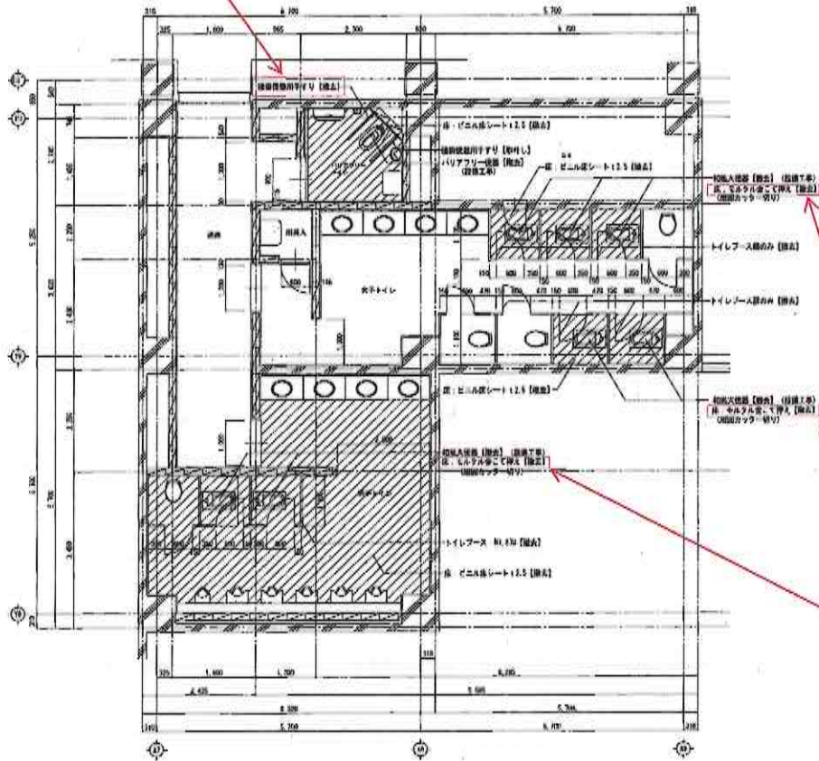
改修前 2階ホールエリア X7-X9間トイレ配り平面詳細図 1/50
