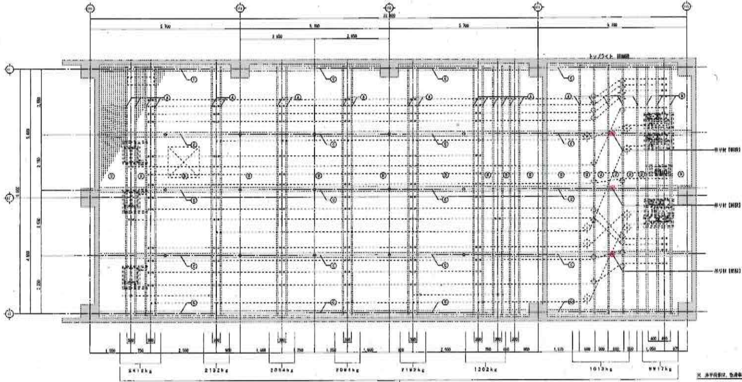
ブドウ棚 伏図 1/20
