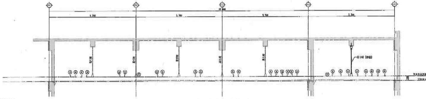
ブドウ棚 側面図 1/20
