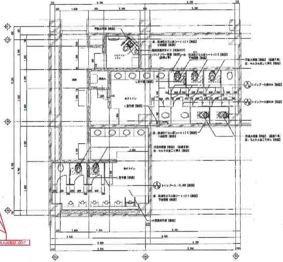
改修後 2階ホールエリア X7-X9間トイレ配り平面詳細図 1/50
