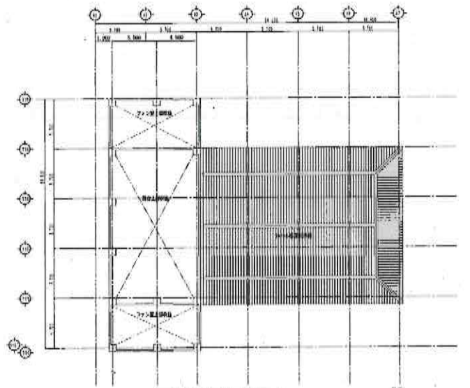
舞台上部平面図 1/200
