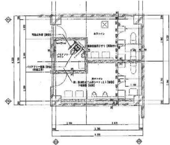
改修後 1階ホールエリア X14-X15間トイレ廻り平面詳細図 1/50
