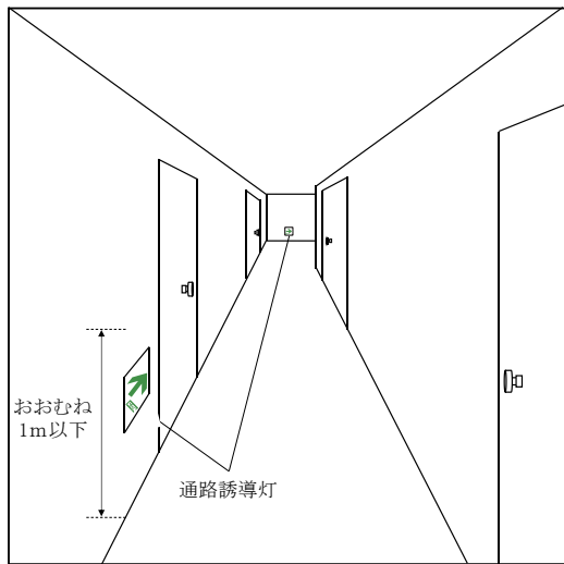
< (2) 項ニ等の通路誘導灯の設置例 >
