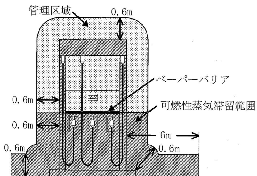
図第 2-1-12 地上式固定給油設備等（可燃性蒸気流入防止構造）
