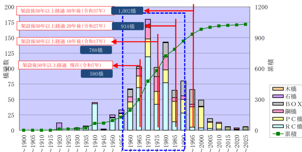
図 1-3 建設年度の分布
