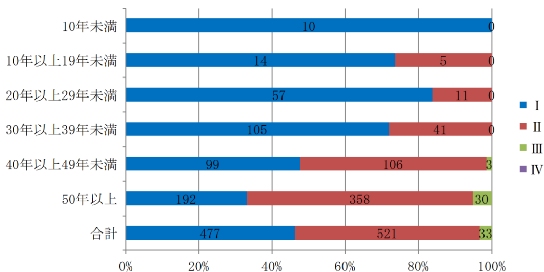
図 5-2 診断区分と建設経過年数
