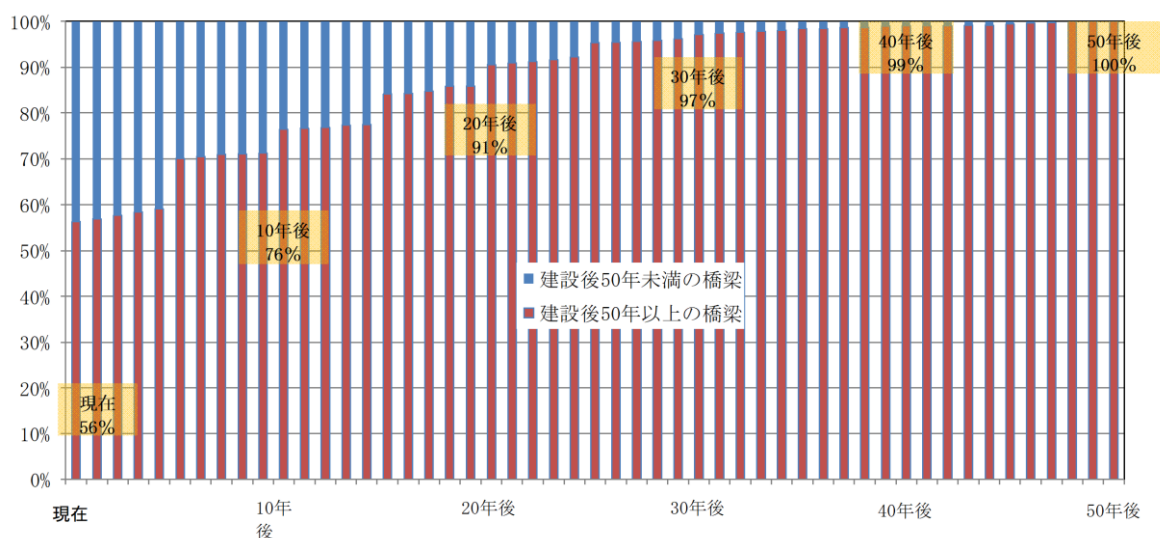
図 1-4 建設後 50 年以上の橋梁数比率
