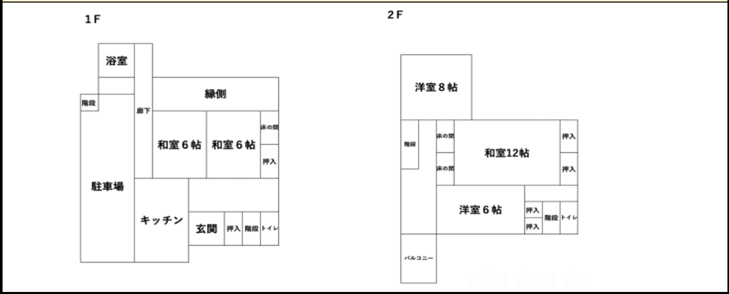
間取図
