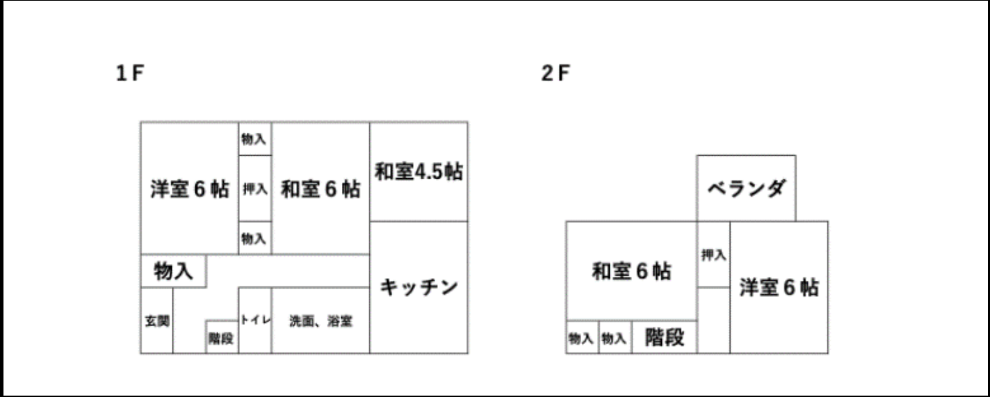
間取図
