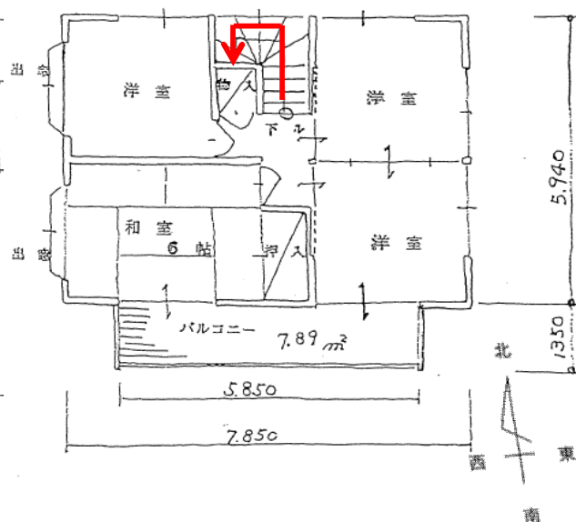
間取図
