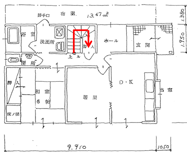
間取図
