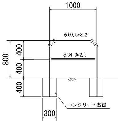
防止柵撤去 縮尺=1:20
