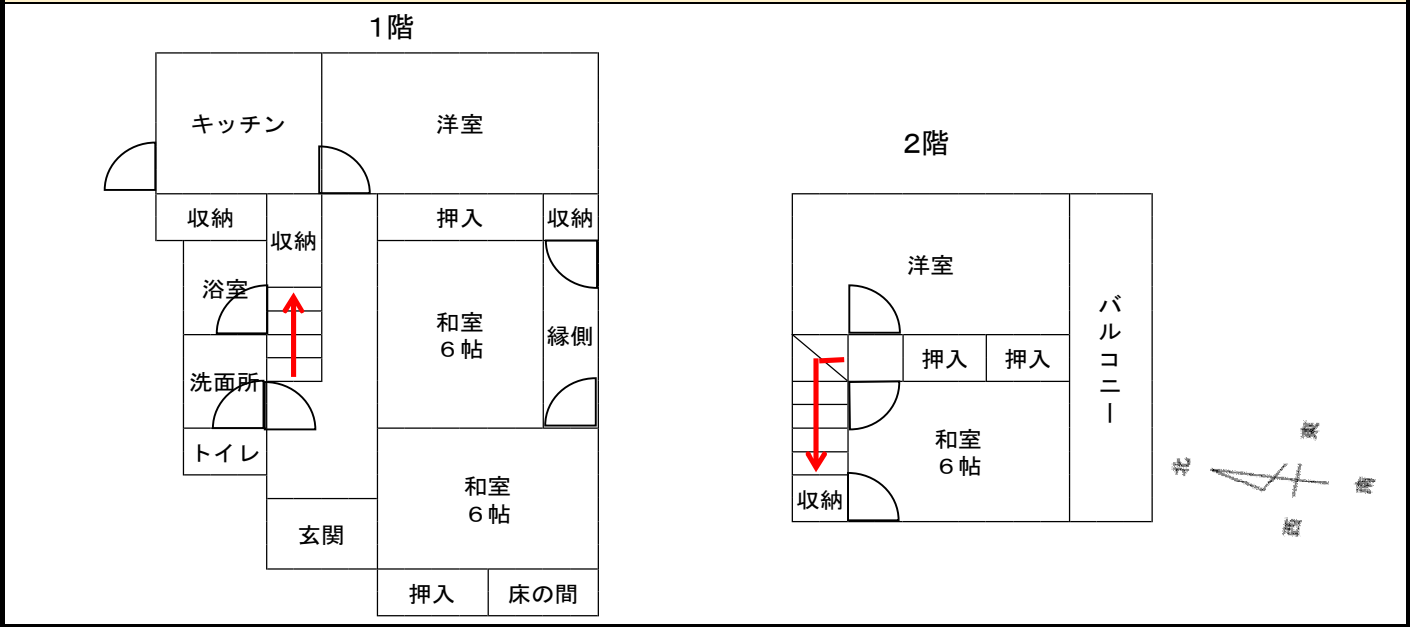
間取図
