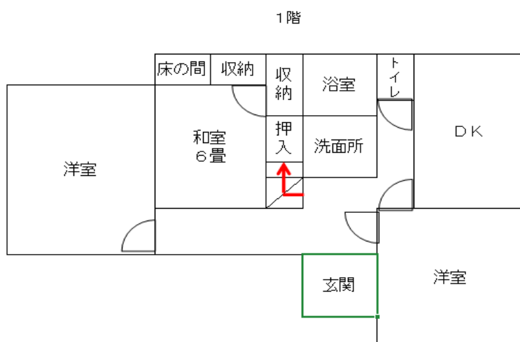
間取図
