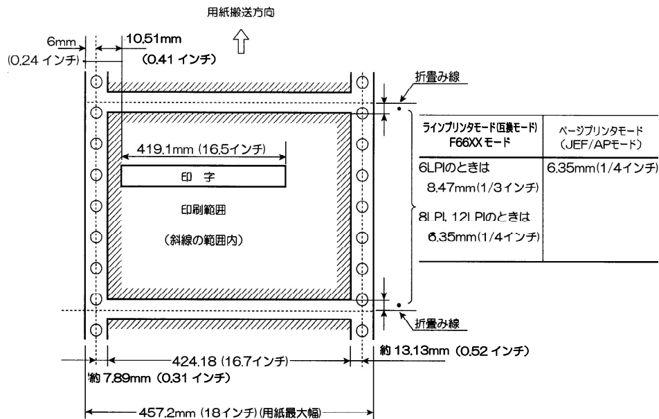
図 3.1 印刷可能範囲 (2/2)
