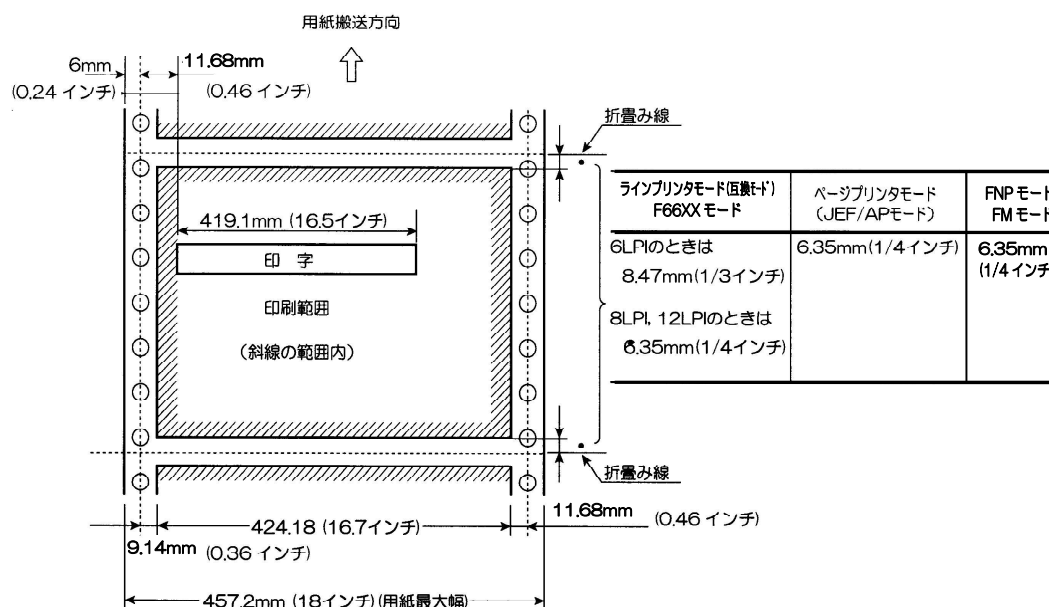
図 3.1 印刷可能範囲 (1/2)
