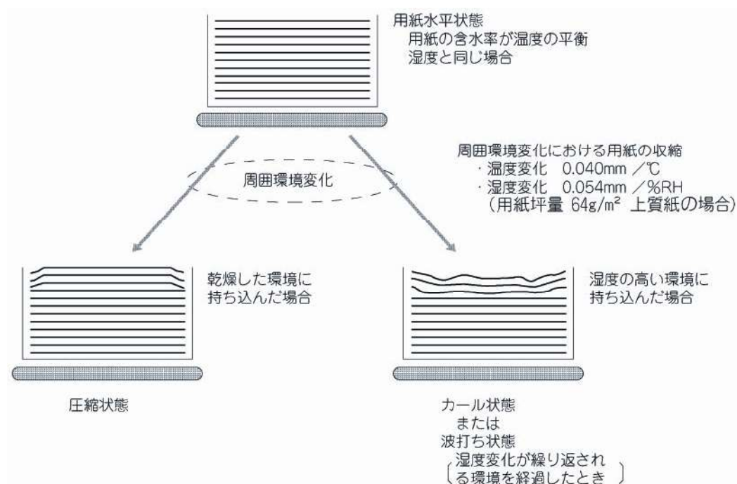
図 3.12 水分量変化による用紙のカール
