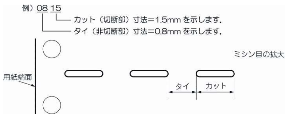
図 3.5 ミシン目の表示寸法
