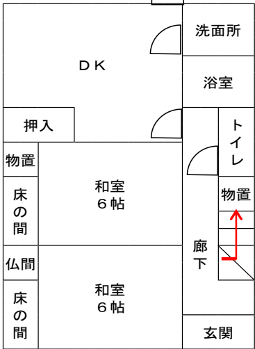
間取図
