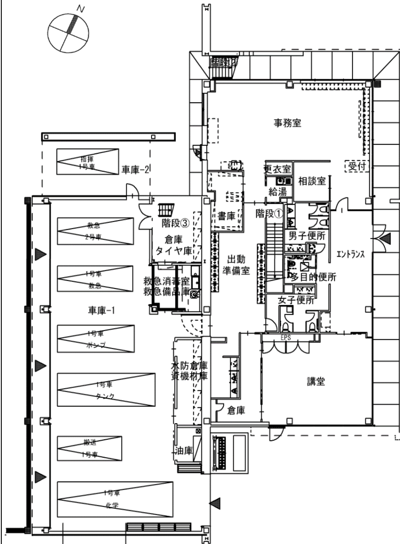
【庁舎棟1階平面図】
