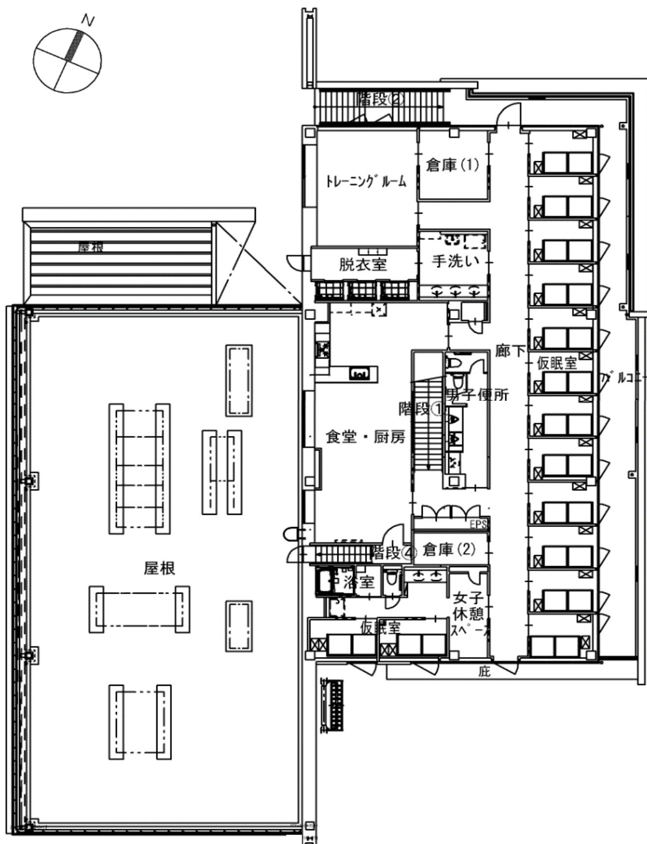
【庁舎棟2階平面図】
