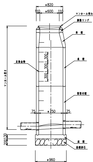
①-①断面
