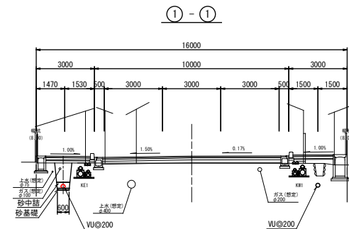
横断面図 S=1/100
