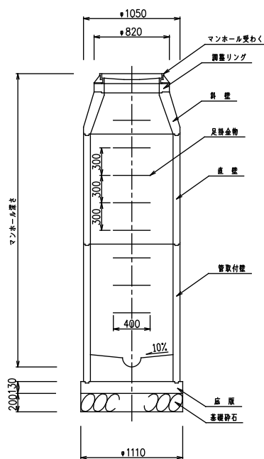
②-②断面
