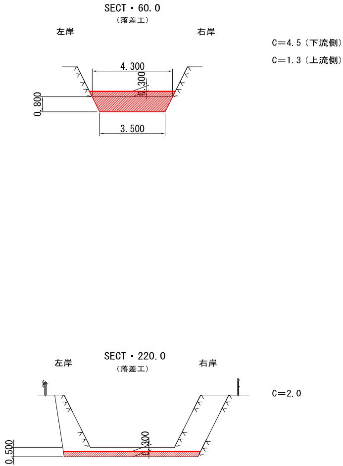
横 断 図
