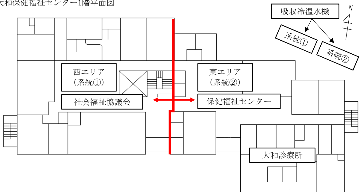
大和保健福祉センター1階平面図
