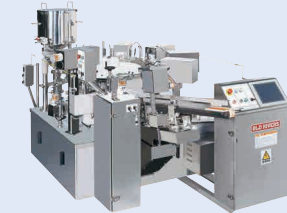
袋詰工程を自動化するシール機
