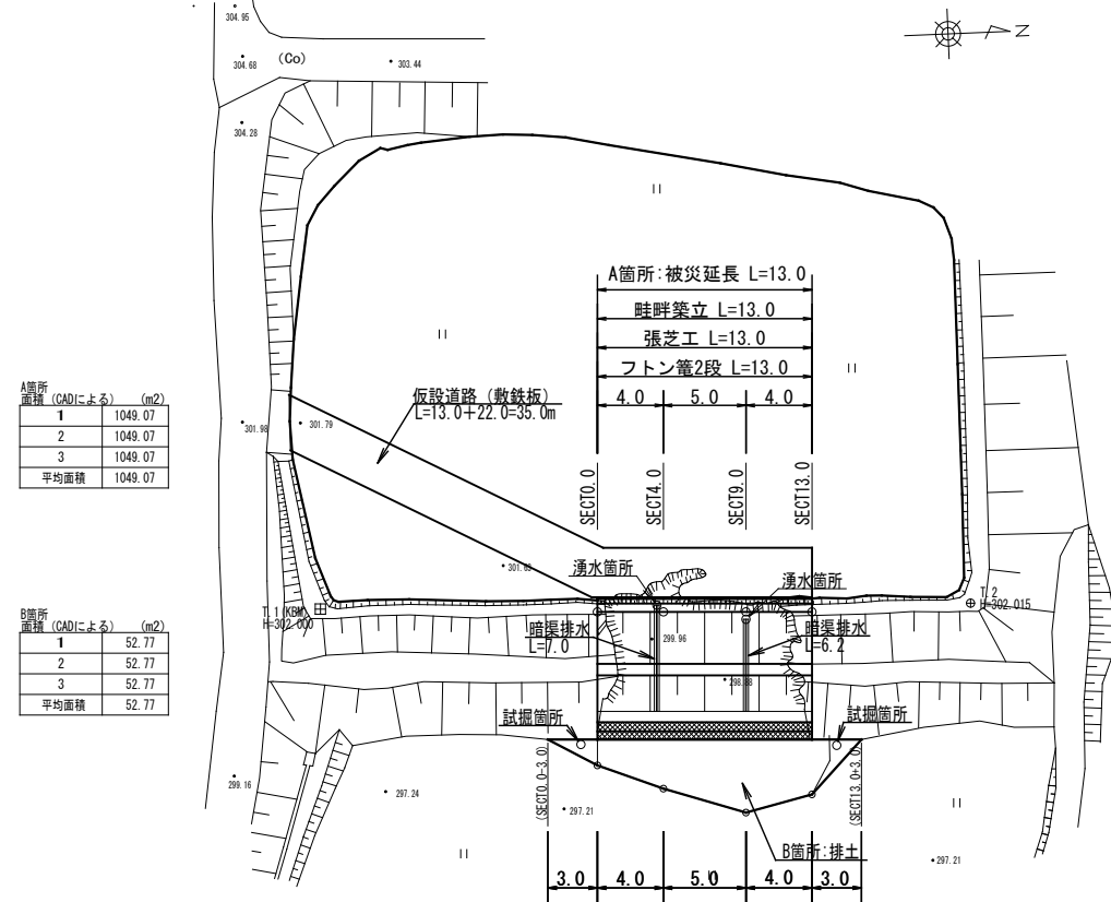
平面図 S= 1:250
