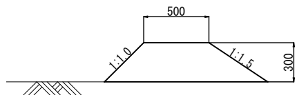
畦畔築立 S=1:20
