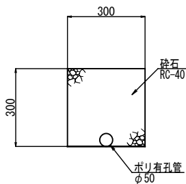
暗渠排水 S=1:10
