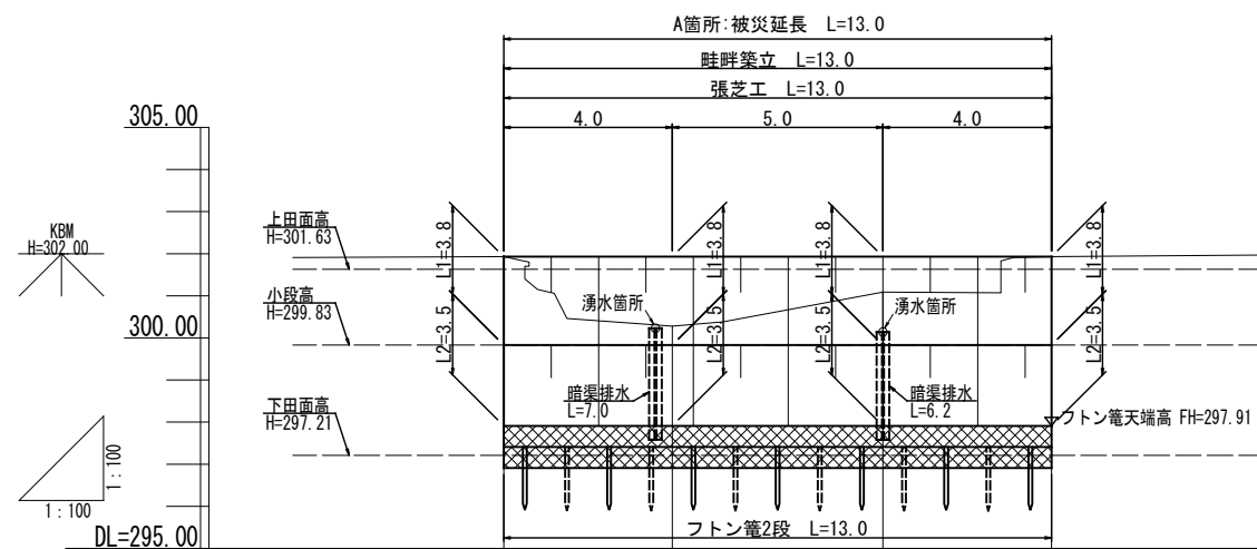
縦断図 V= 1:100 H= 1:100
