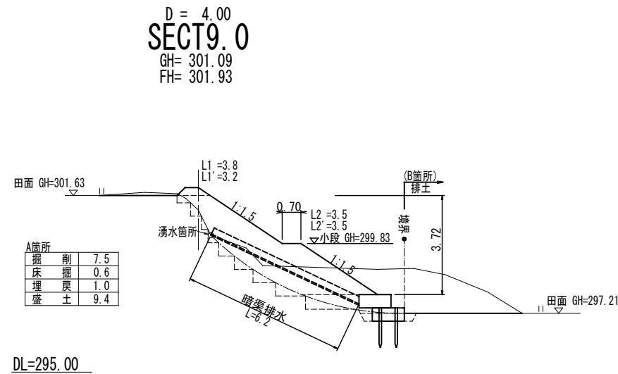
A箇所 横断図 S=1:100
