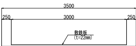
仮設道路（敷鉄板）
