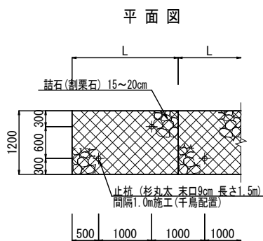
フトン簀 S=1:50
