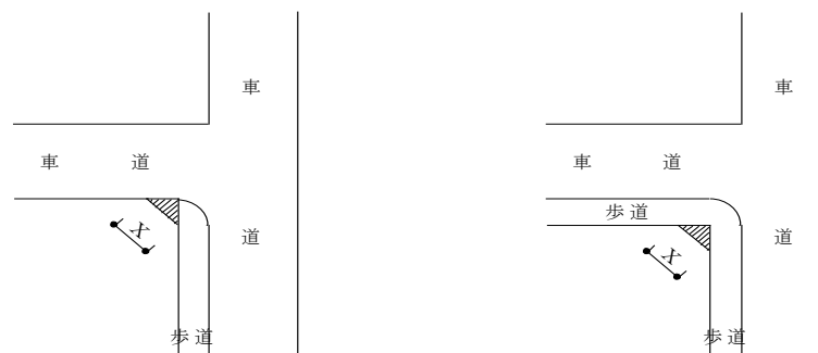
歩道を有する場合の隅切寸法(X)の取り方
