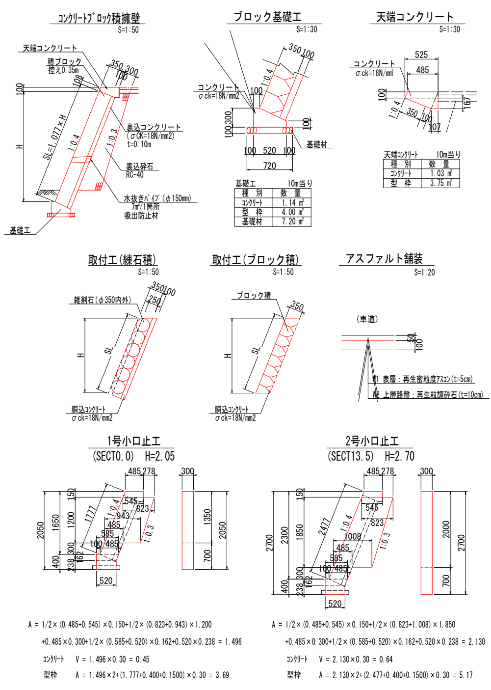
構造図 縮尺=図示
