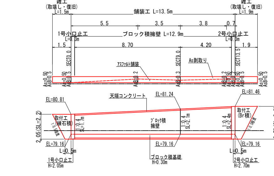
構造図 縮尺=図示
