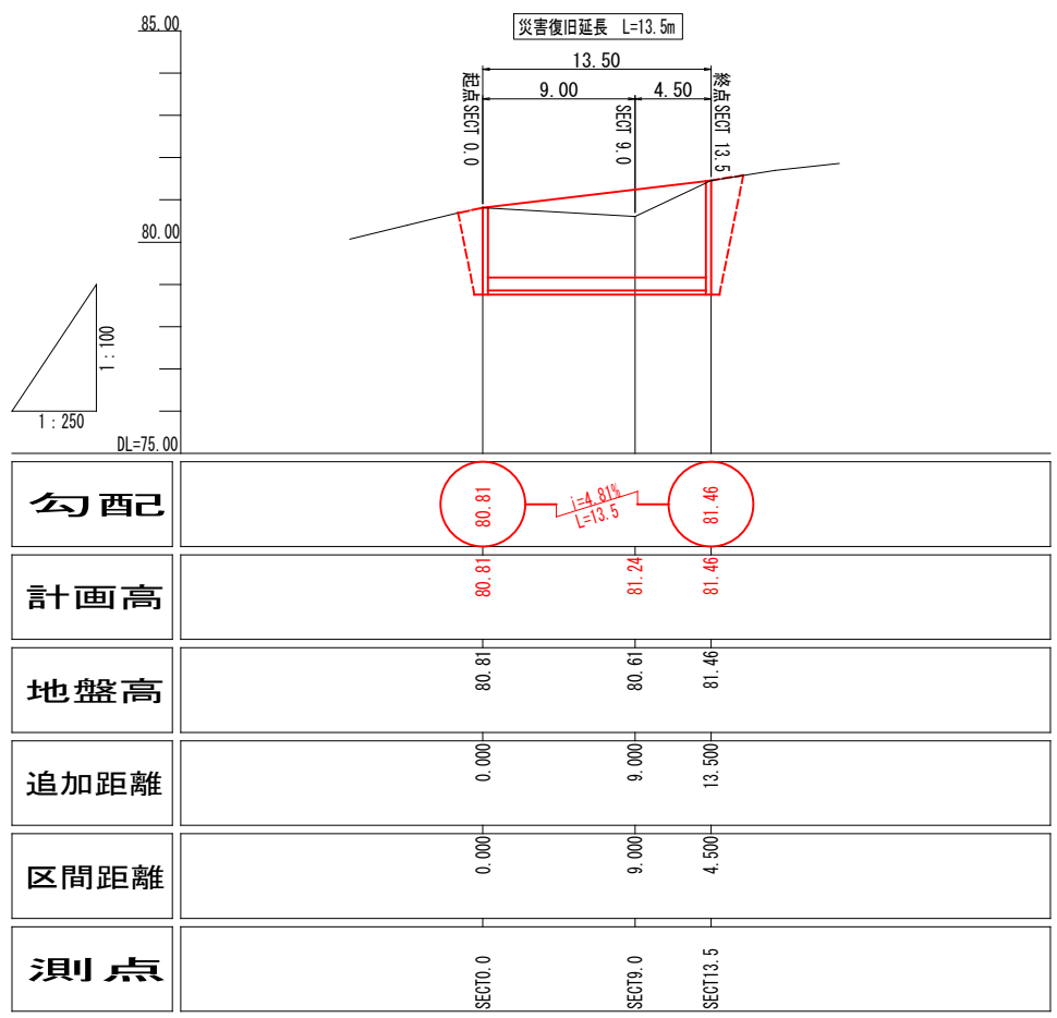
縦断面図 縮尺= V=1:100 H=1:250
