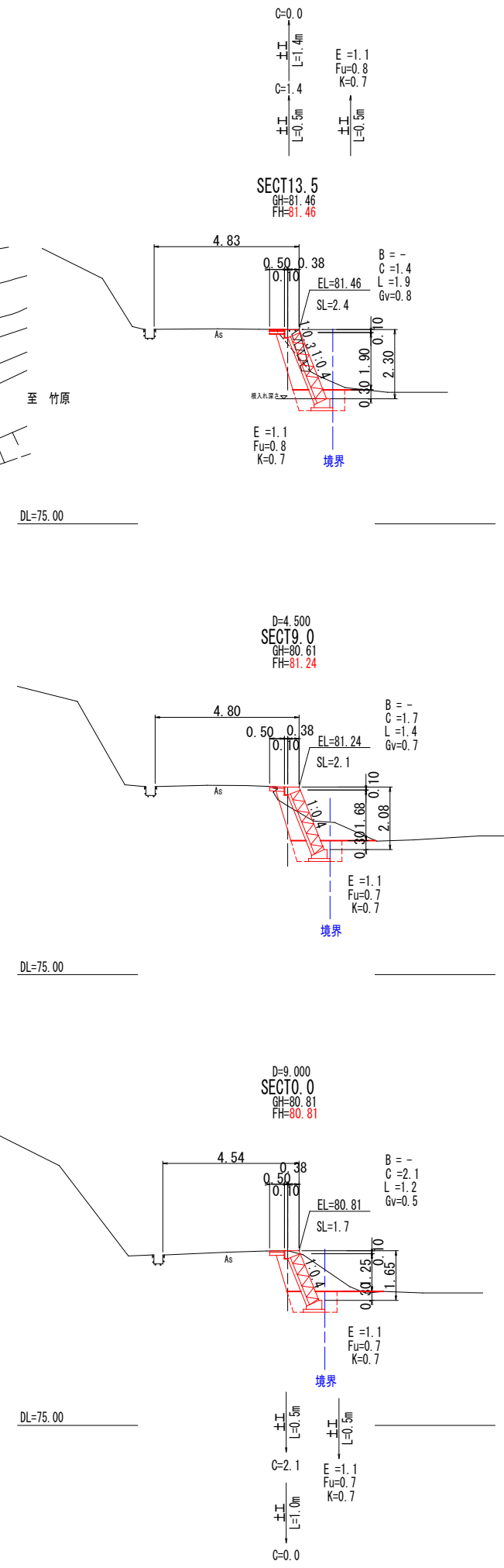
横断面図 縮尺=1:100
