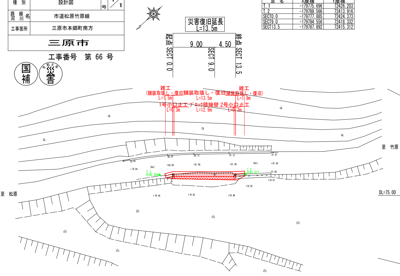
平面図 縮尺=1:250
