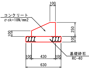
ブロック基礎 S=1:20
