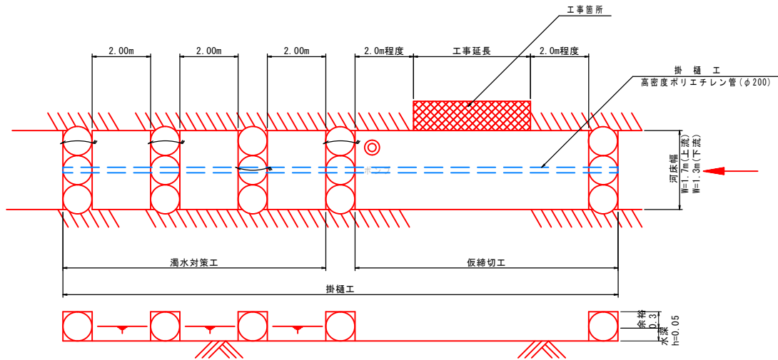
(参考図) 大型土のう標準図 S=1:100 (河床幅3m未満)
