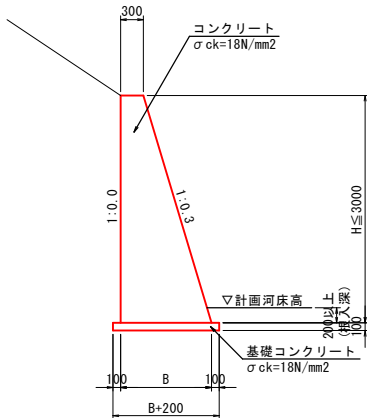
断面図 S=1:50
