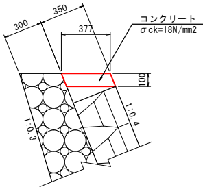
天端コンクリート S=1:20
