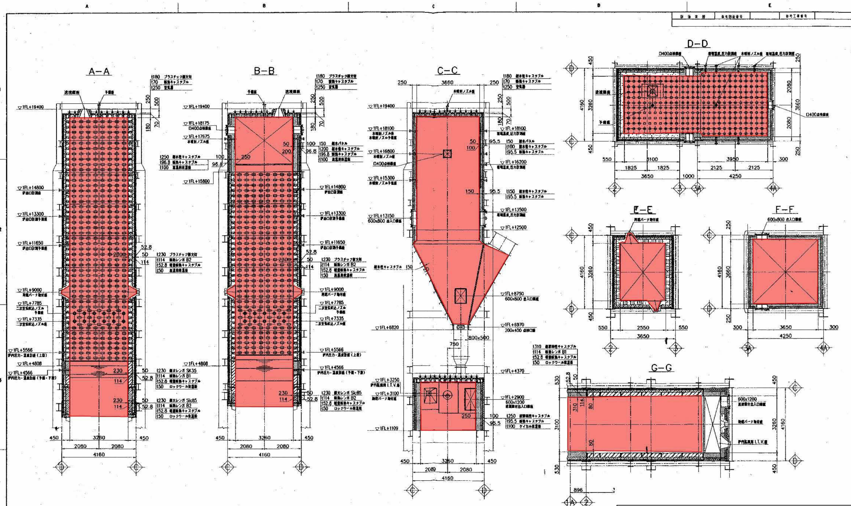
三原市清掃工場 2号炉クリンク除去範囲図②
