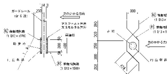
鉄筋組立図
