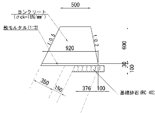
支柱基礎部詳細図
