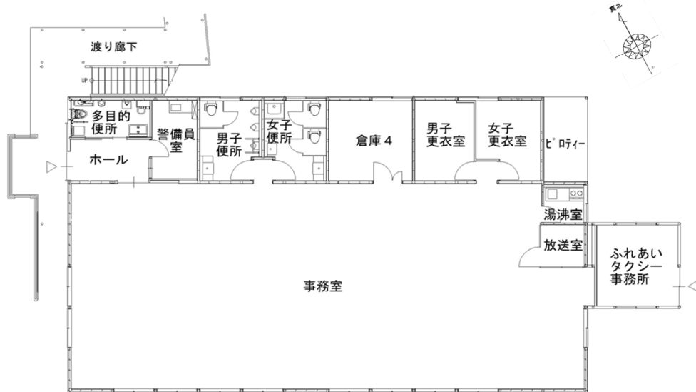
1階平面図
