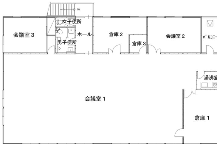
2階平面図
