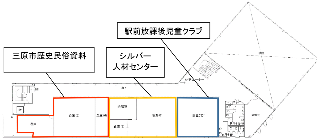
2階平面図
