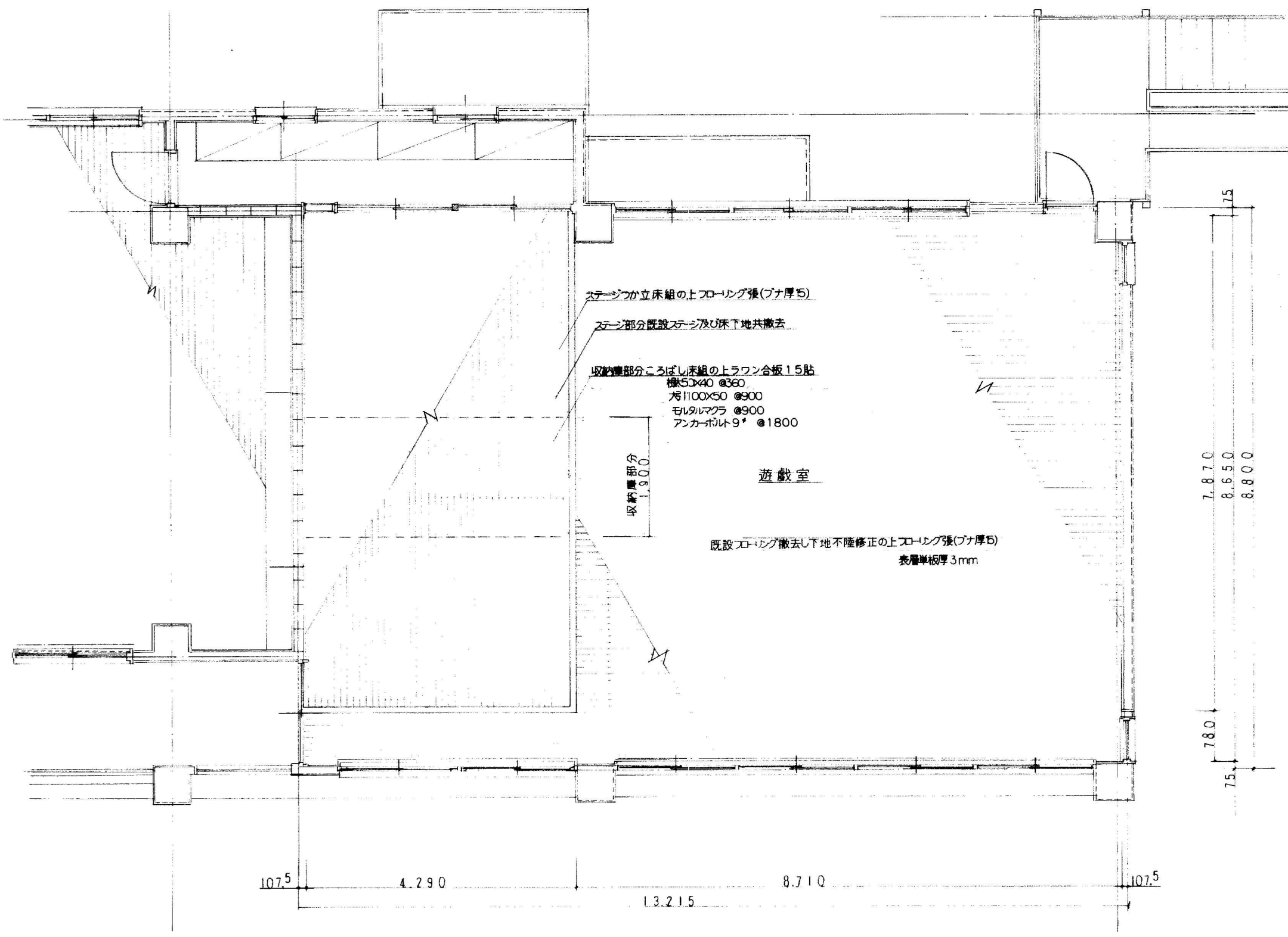
平面図 縮尺 1:50
