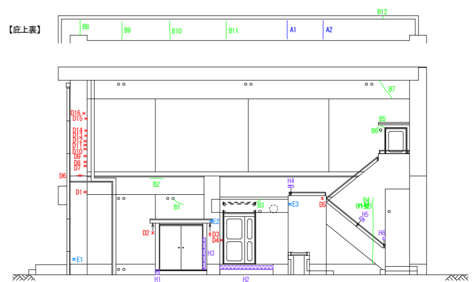
西立面図
