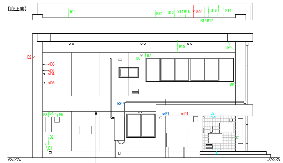
東立面図
