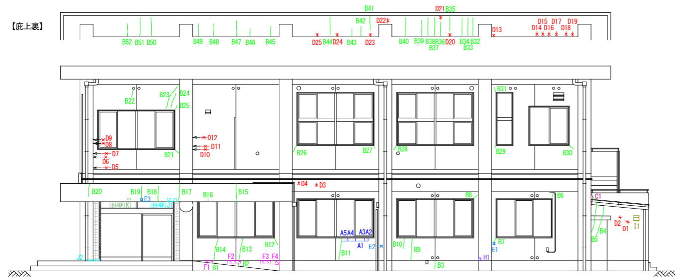
北立面図
