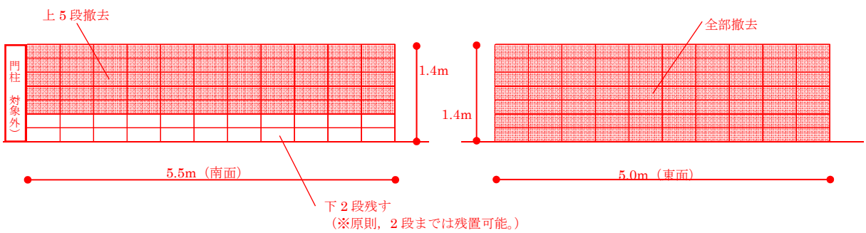
南面 立面図 (現状)
