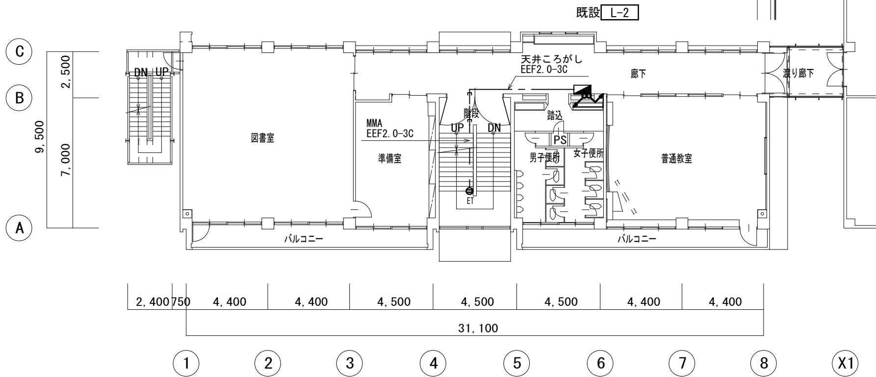
2階平面図 S=1/200
