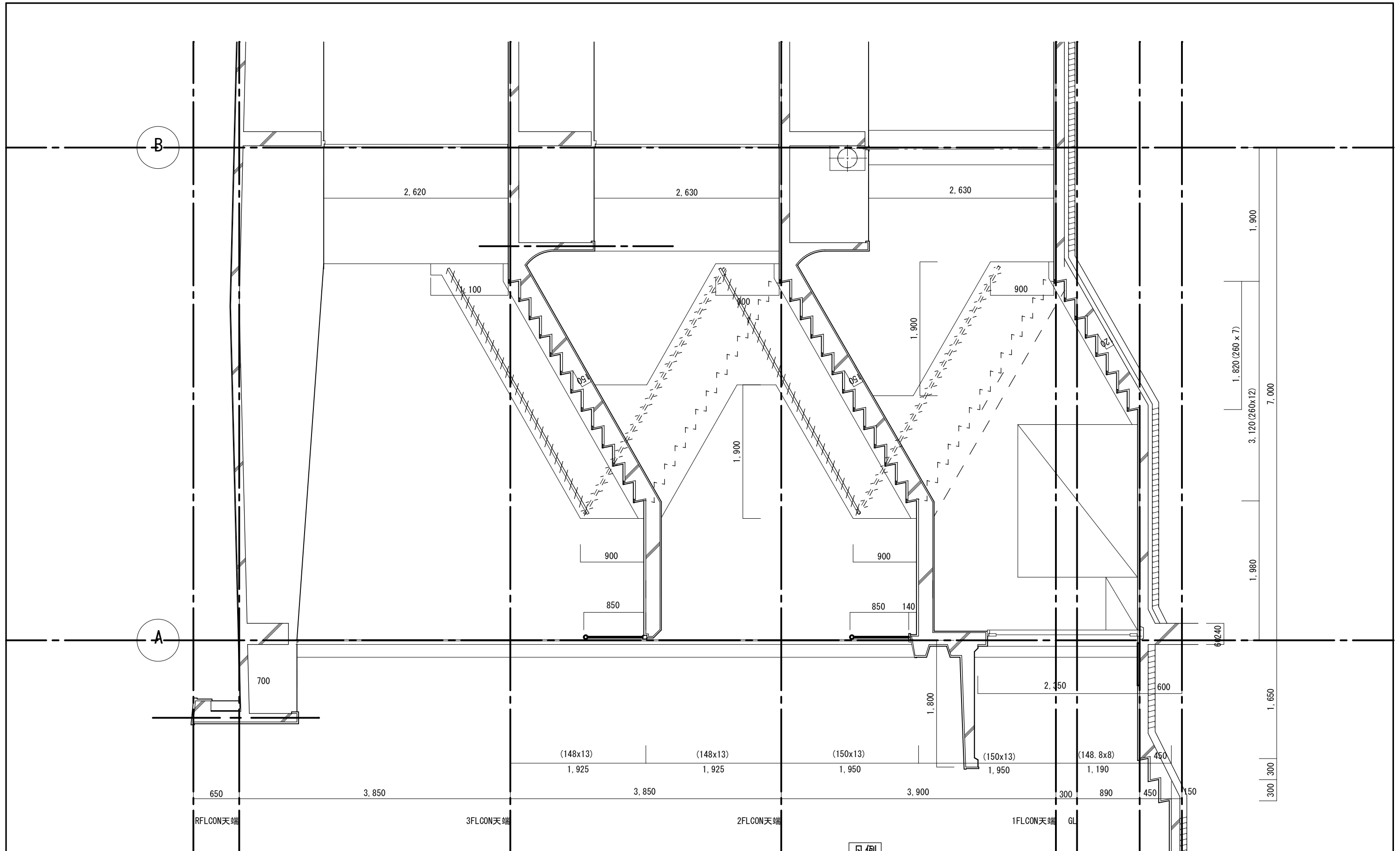
階段 断面詳細図 S=1/50
