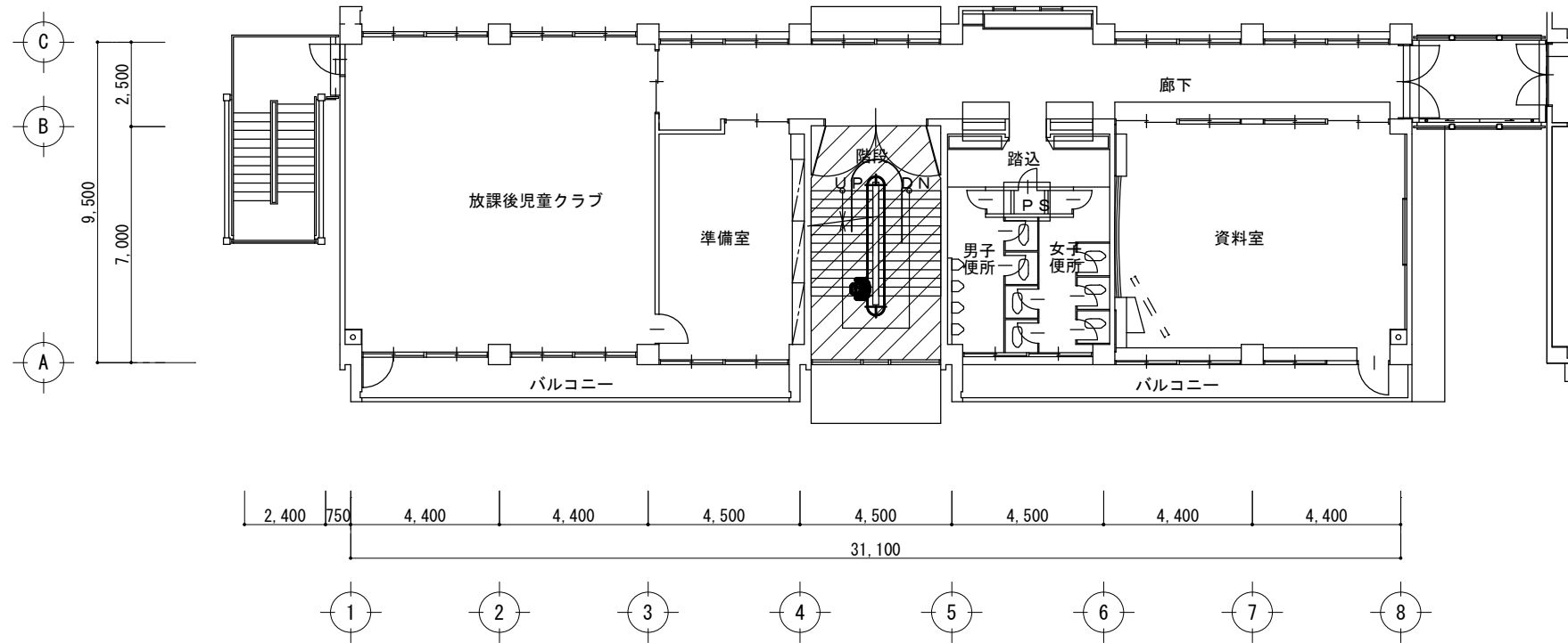
2階平面図 S=1/200
