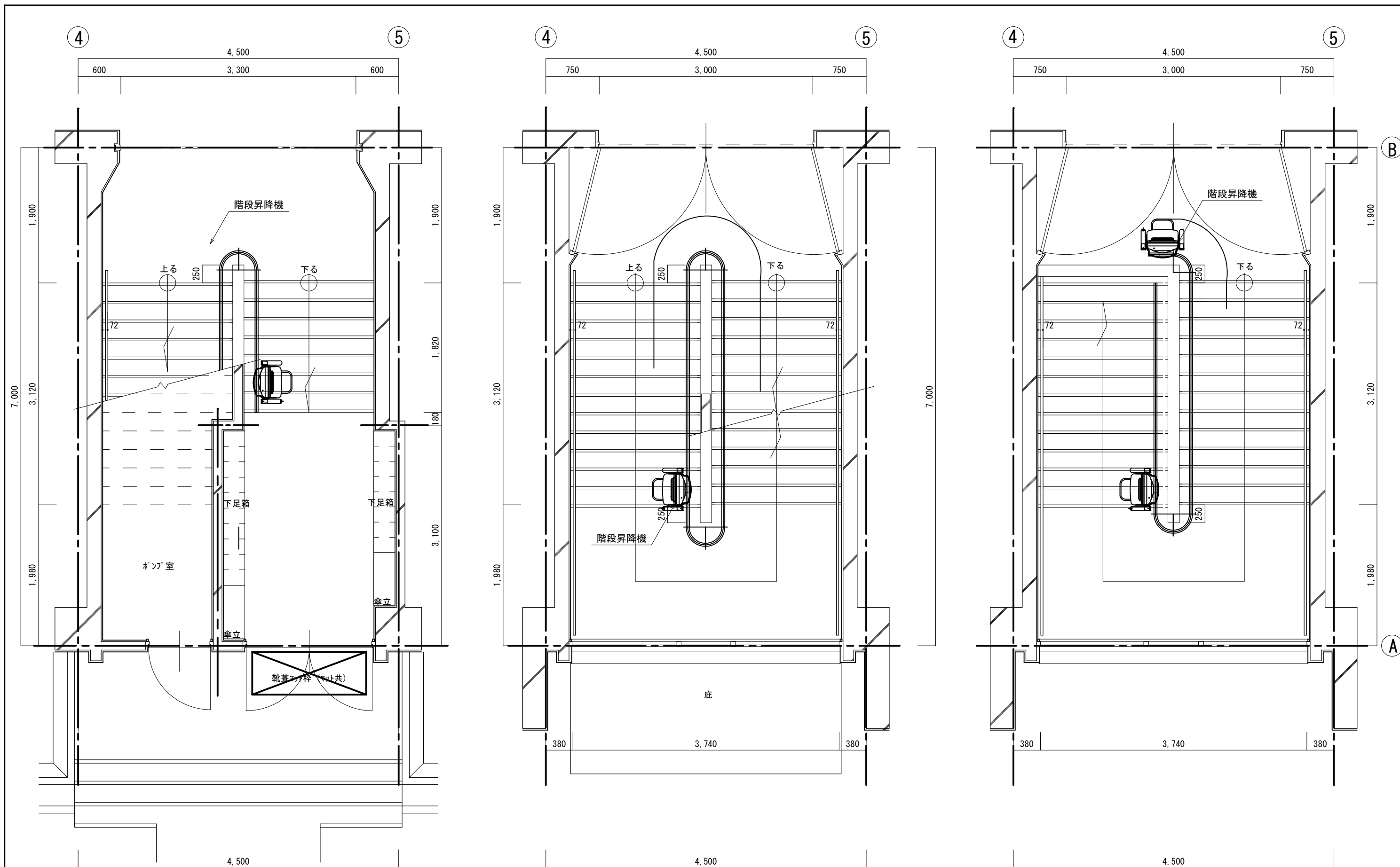
1階 階段平面詳細図 S=1/50
