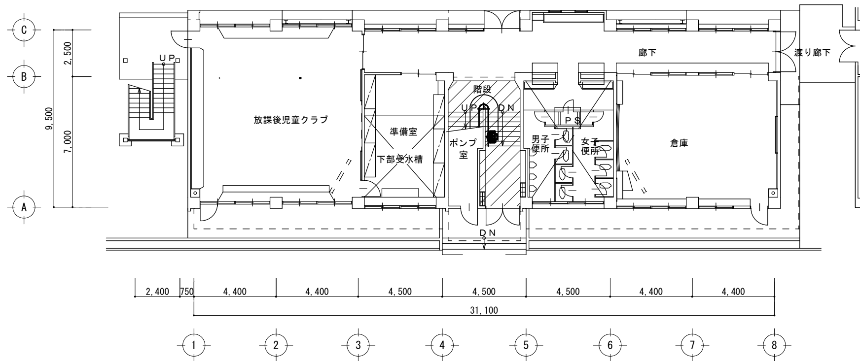
1階平面図 S=1/200
