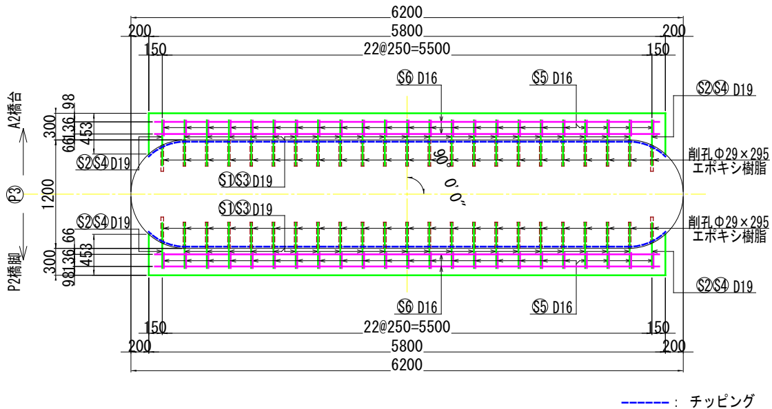
鉄筋加工図
