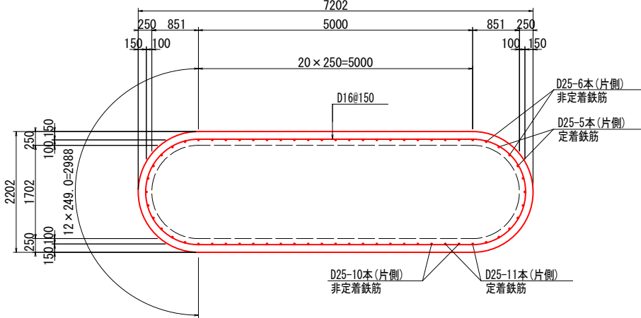
補強断面図 柱基部
