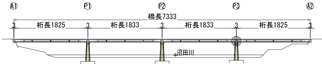
位置図
