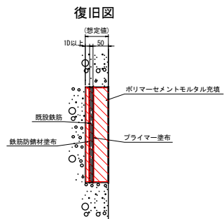
断面修復工詳細図 (左官工法)
