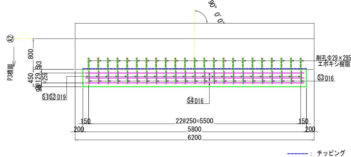
平面図 S=1:30
