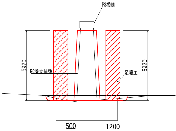
橋脚部 足場工断面図 S=1:100
