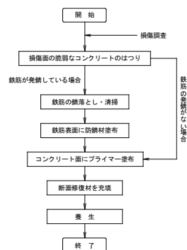
施工フロー
