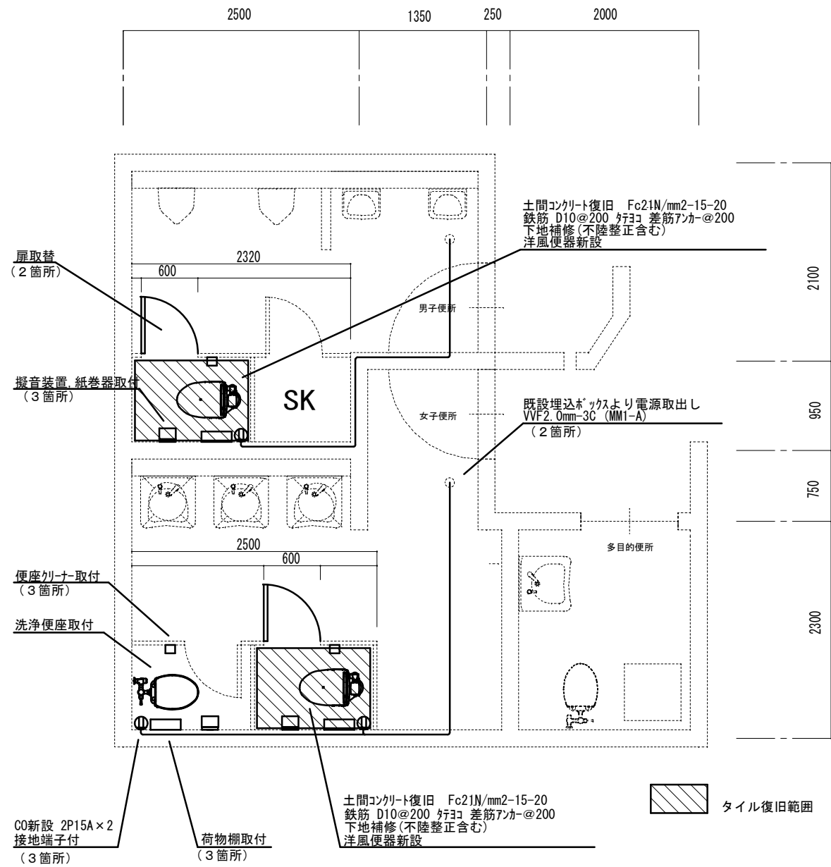
平面詳細図 改修後 S=1/40
