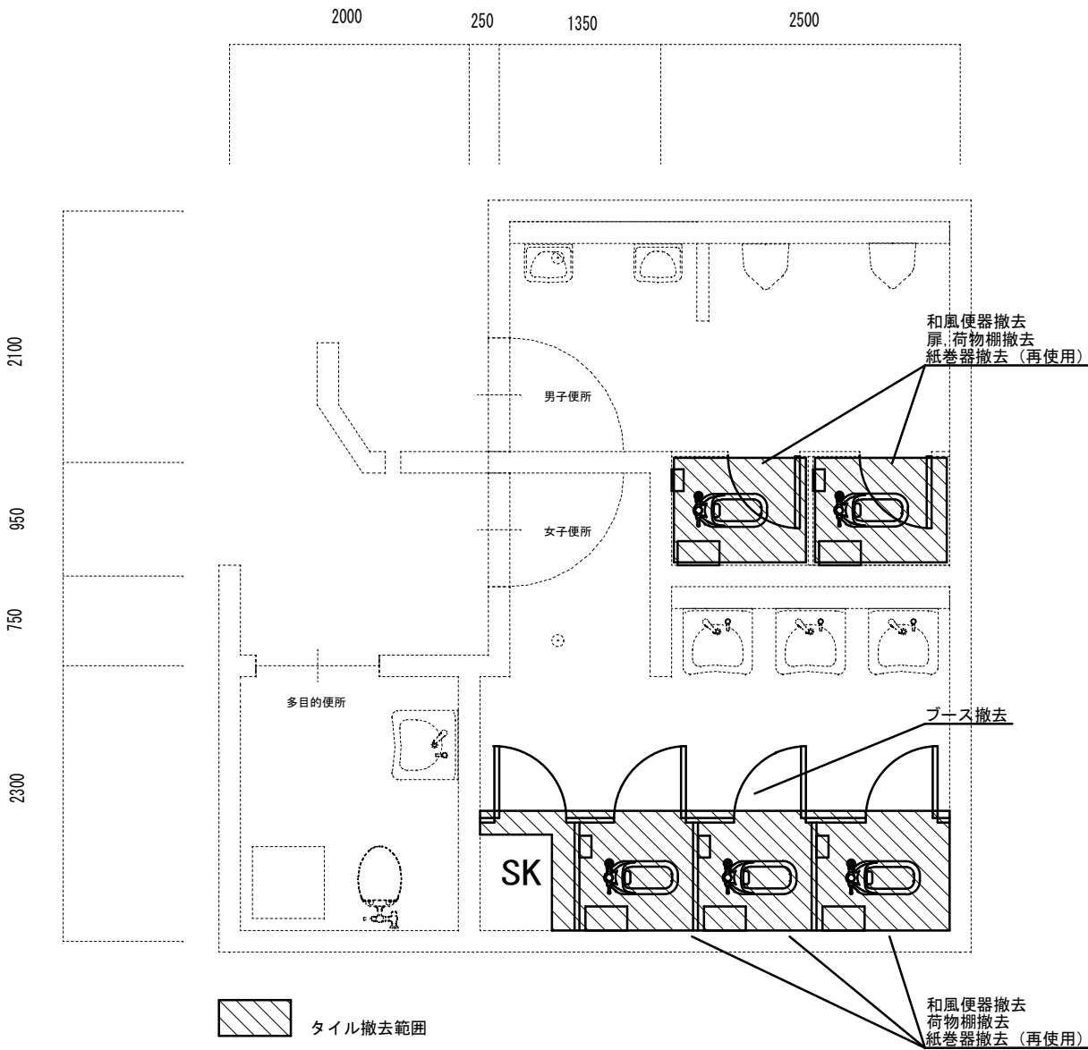
平面詳細図 改修前 S=1/40
