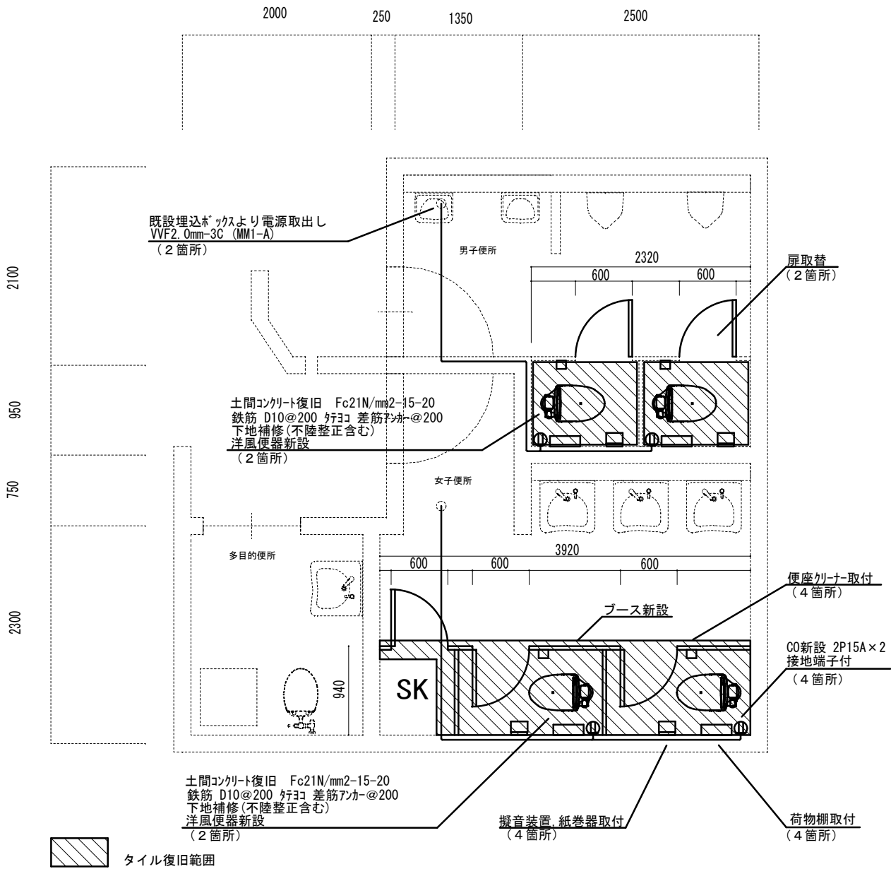
平面詳細図 改修後 S=1/40
