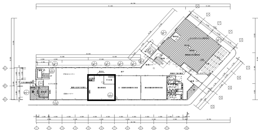
1階 平面図
