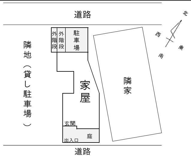
配置図
