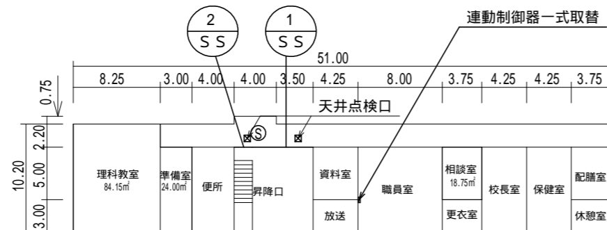
9 1階
