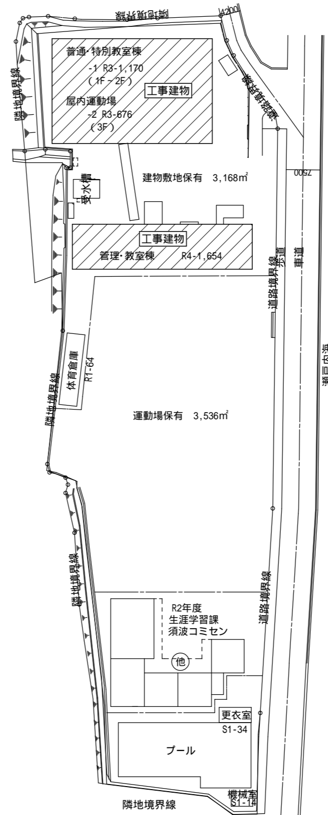
配置図 S=1/800
