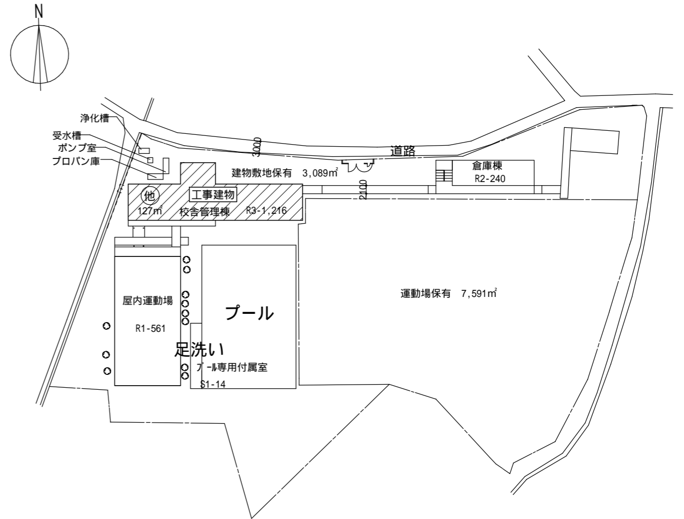
配置図 S=1000
