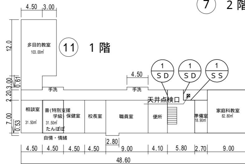
7 1階
