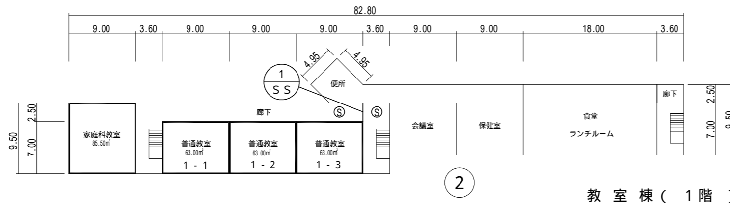
教室棟 ( 2階 )
