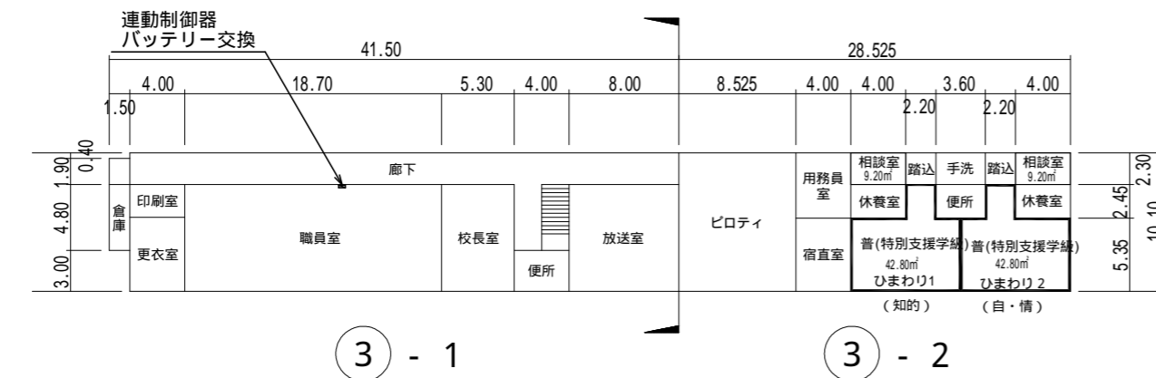
管理棟・教室棟 ( 1階 )
