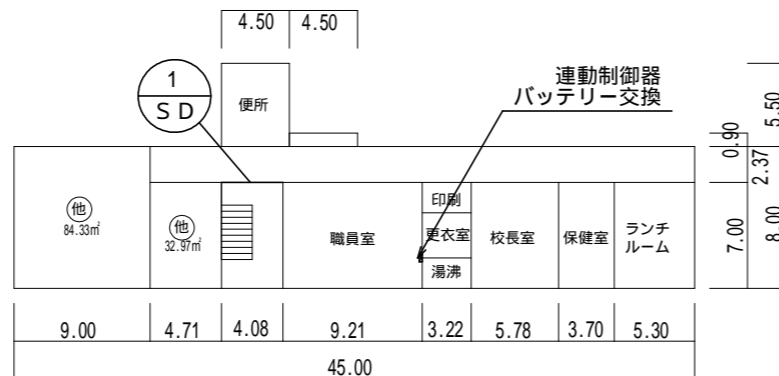
⑧ 1階
