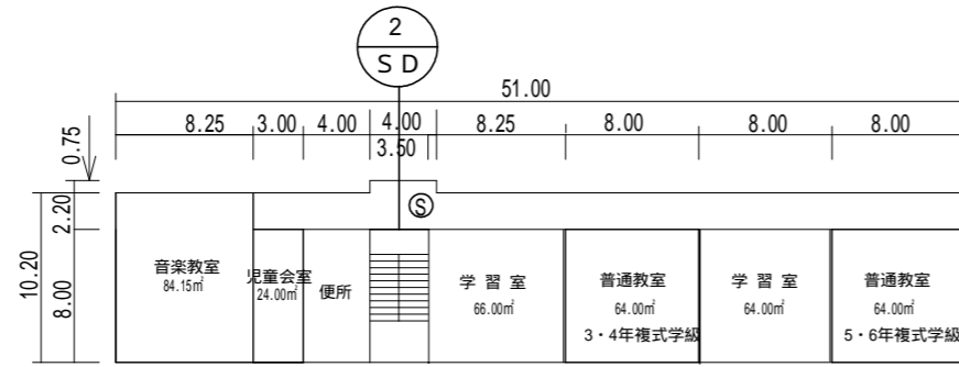
9 3階
