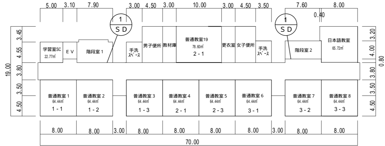
① - 2階
