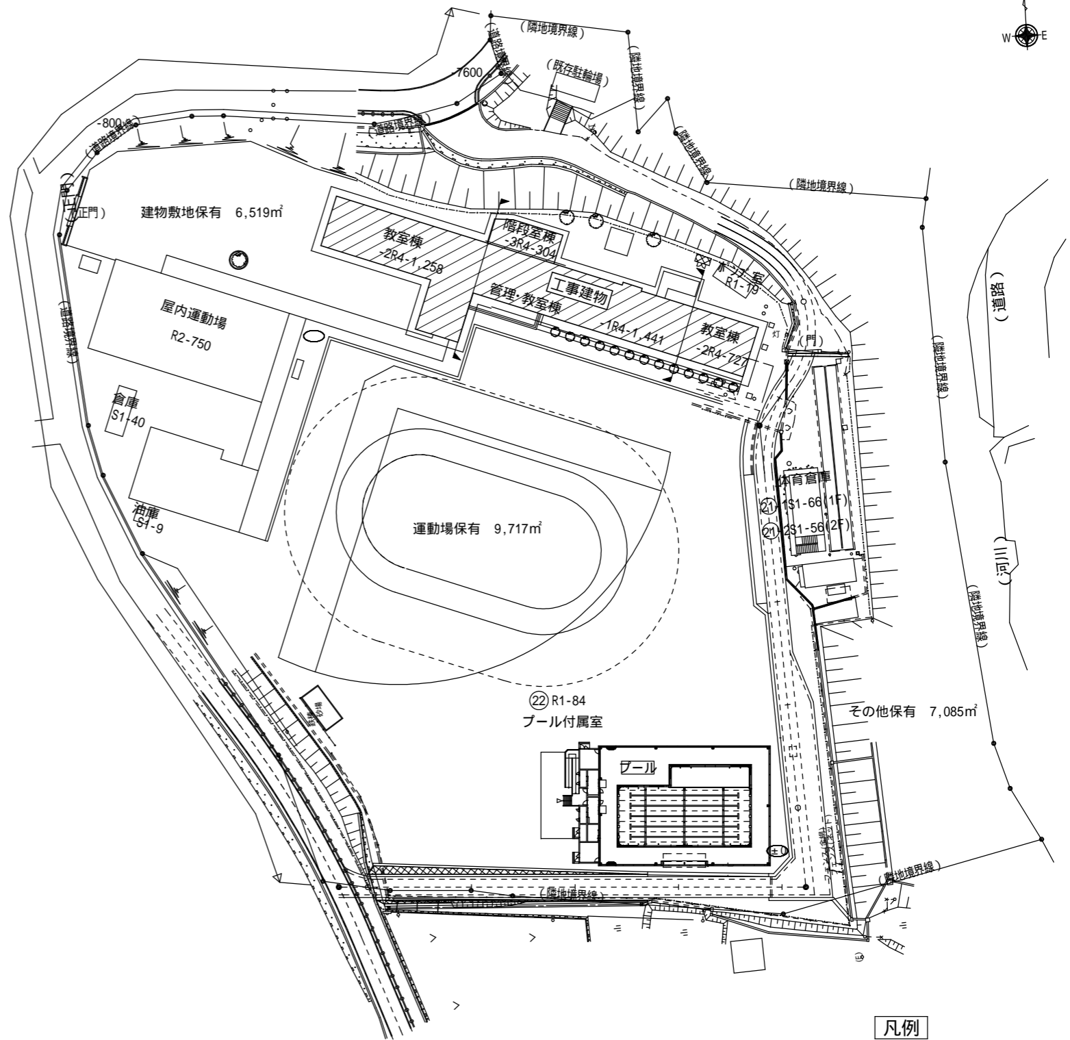
配置図 S=1/1000
