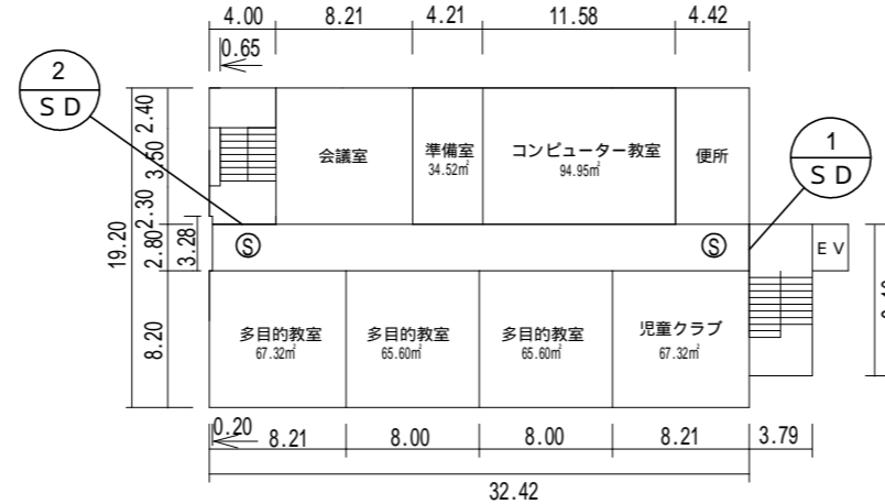
2階 11 - 1
