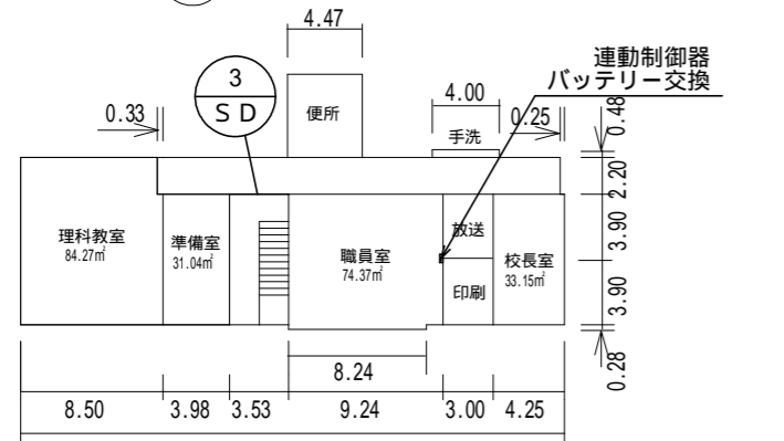
1階 9
