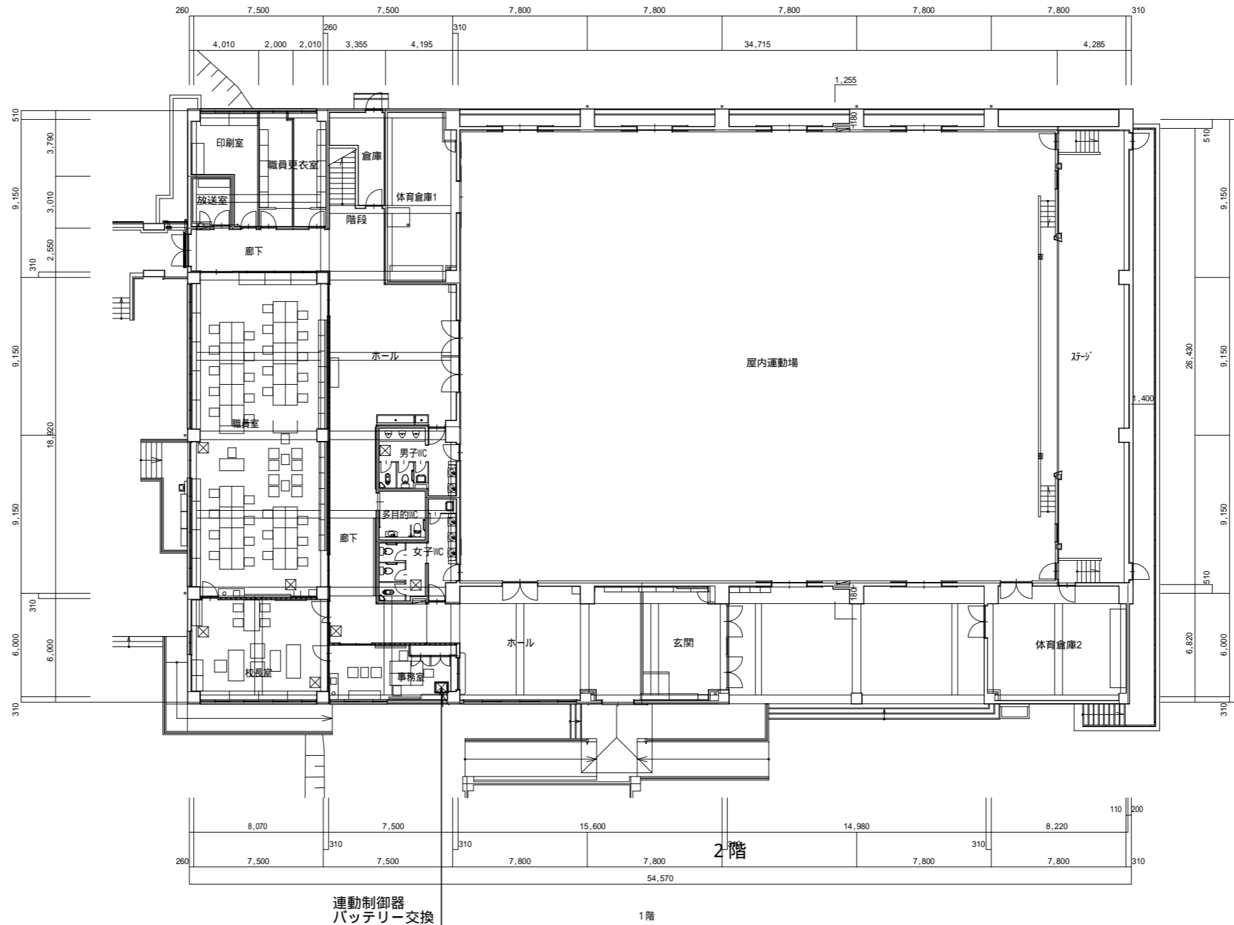
1階平面図 S=1/300
