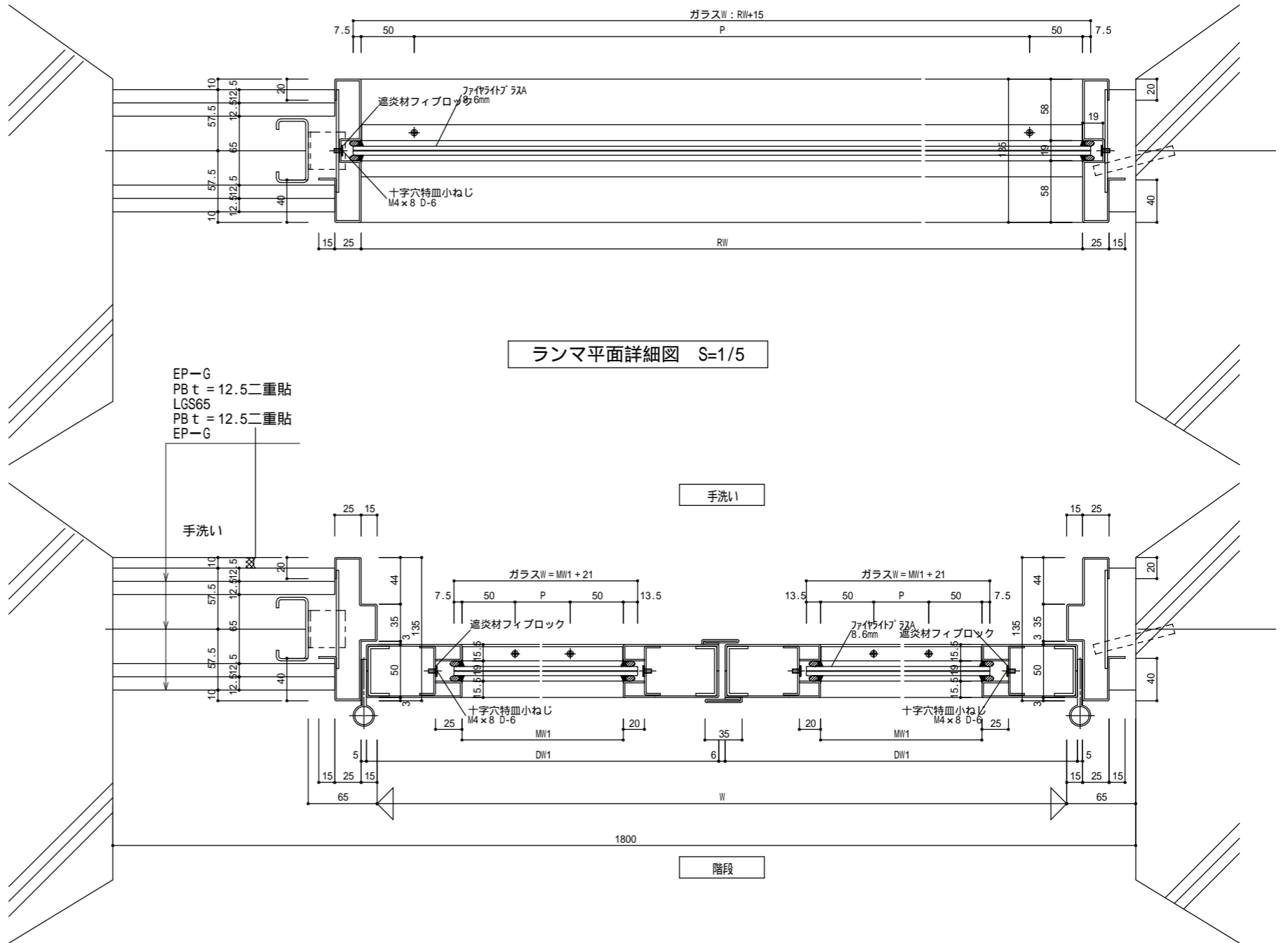
建具平面詳細図 S=1/5
